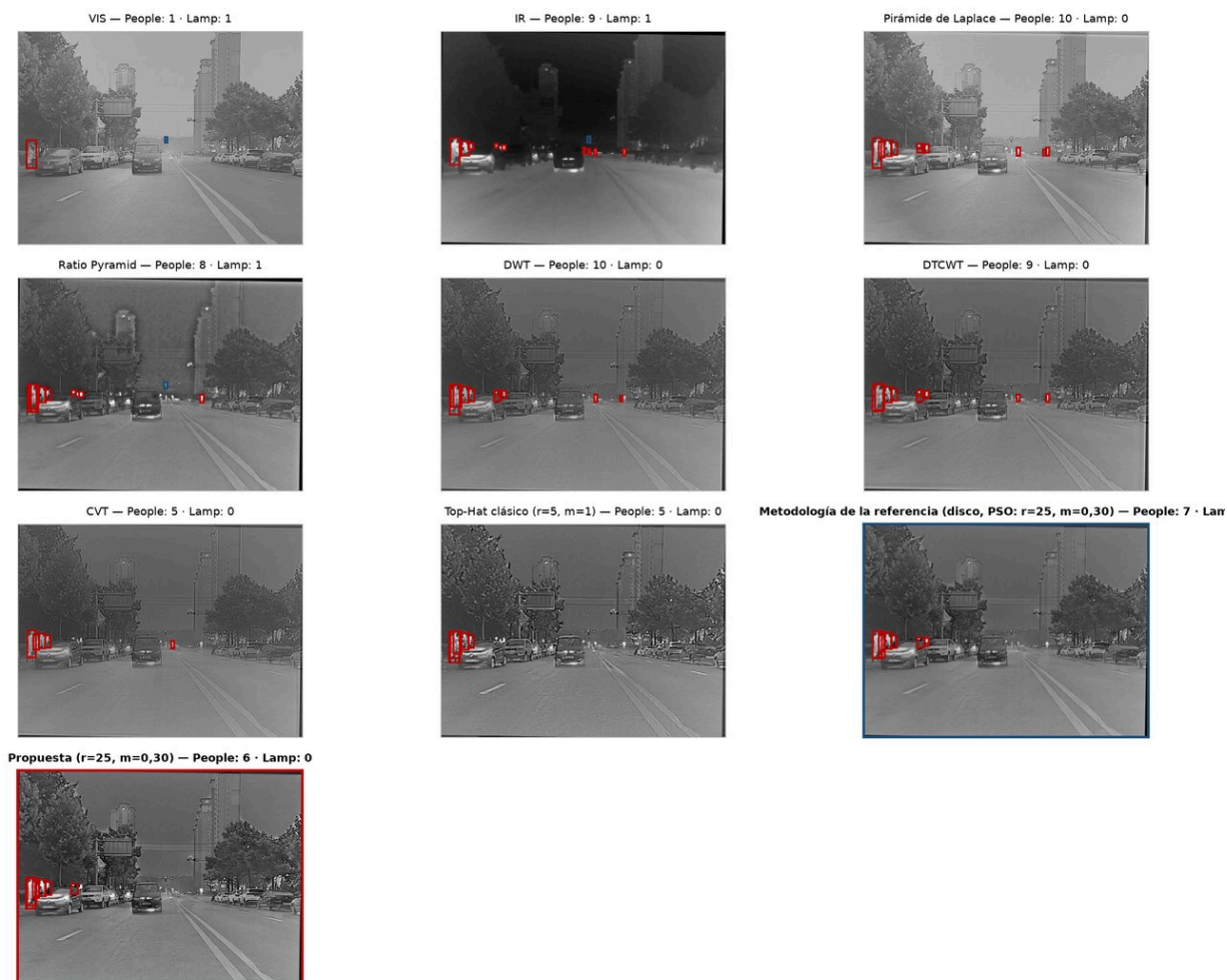
Figura 11. M3FD, escena 00147: detecciones del modelo único VIS+IR sobre las 10 entradas. People en granate, Lamp en azul, umbral de confianza 0,30. Verdad de campo: 12 personas y 1 luz.
