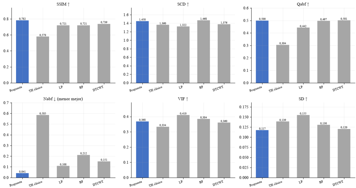
Figura 10. Propuesta Novedosa (PSO: r = 25 , m = 0,30 ) frente a la metodología clásica Top-Hat y al estado del arte en las métricas estándar de calidad.
