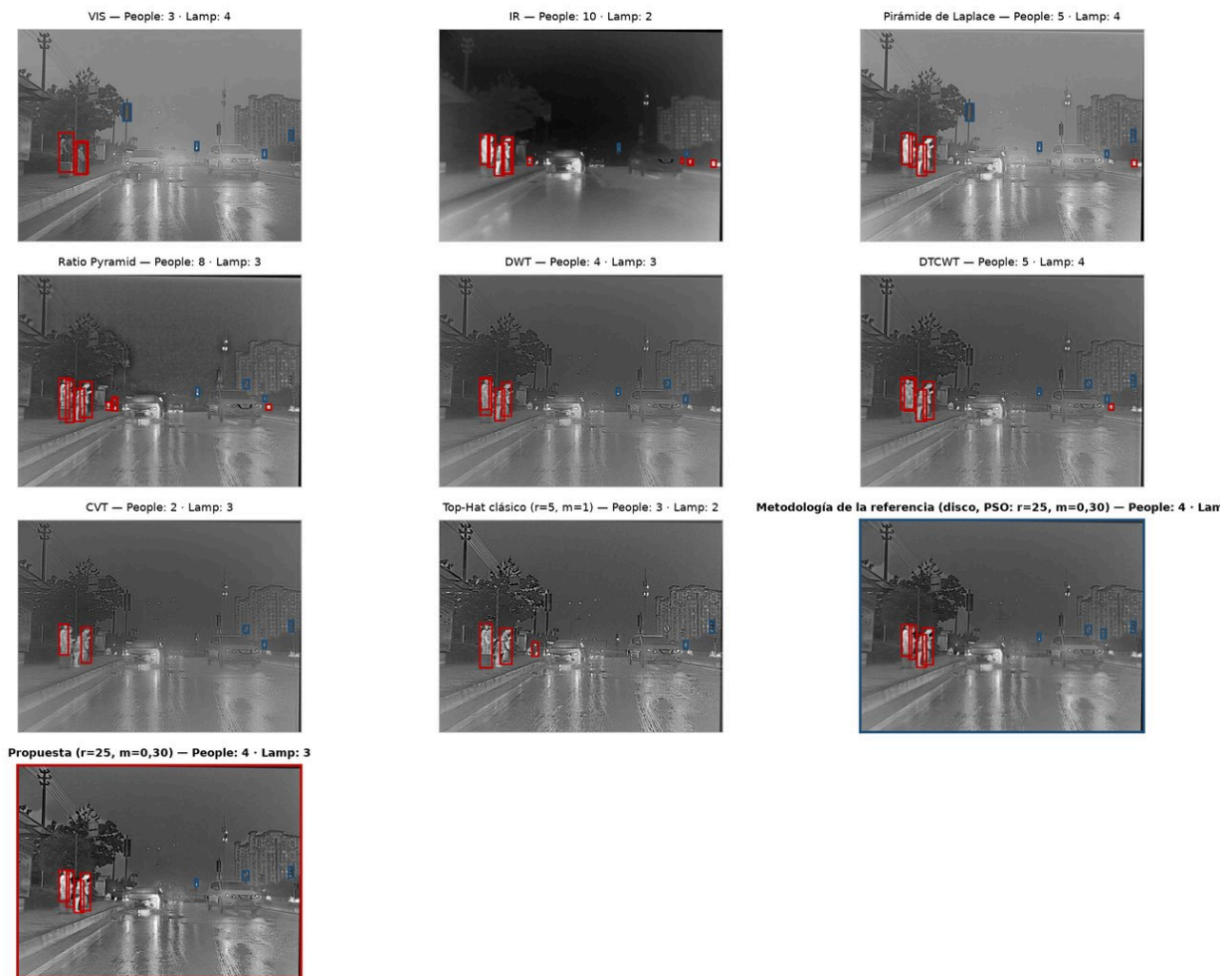
Figura 12. M3FD, escena 00232: detecciones del modelo único VIS+IR sobre las 10 entradas. People en granate, Lamp en azul, umbral de confianza 0,30. Verdad de campo: 12 personas y 6 luces.
