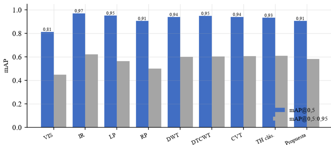
Figura 7. mAP por entrada del detector (YOLOv8n reentrenado por método sobre LLVIP).
