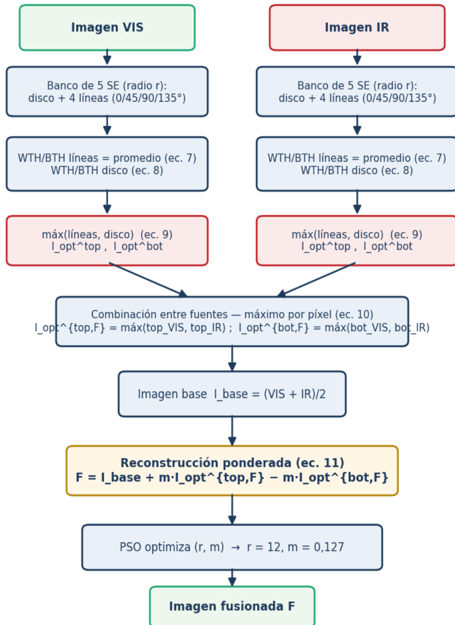
Figura 4. Flujograma de la Propuesta Novedosa: proceso paso a paso (banco de cinco elementos estructurantes por fuente, promediado de las respuestas lineales, suma con la respuesta del disco para obtener las transformadas óptimas, combinación entre fuentes por máximo y reconstrucción ponderada con el peso m ).
