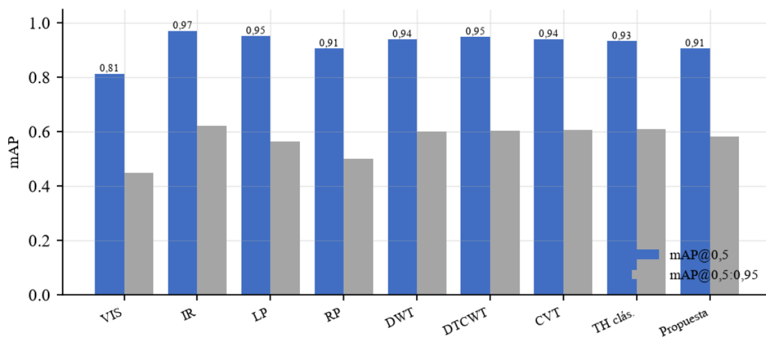
Figura 7. mAP por entrada del detector (YOLOv8n reentrenado por método sobre LLVIP).
