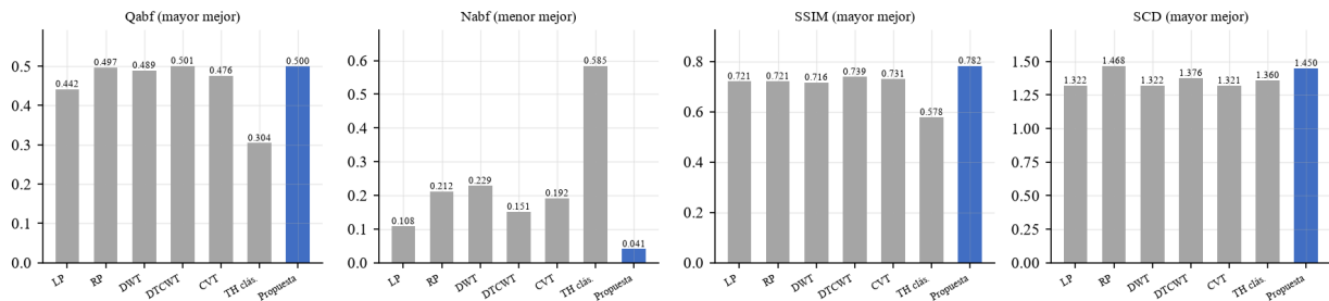
Figura 4. Las cuatro métricas de calidad de fusión; la barra azul es la propuesta.
