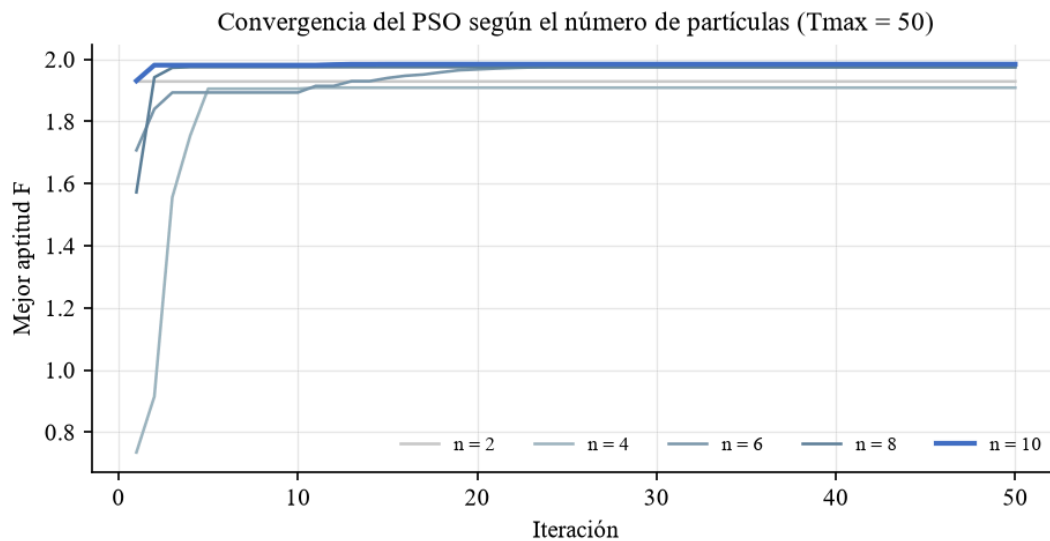
Figura 3. Convergencia del mejor global según el número de partículas (Tmax = 50): los enjambres grandes escapan del óptimo local r = 1 y alcanzan F = 1,9843 .
