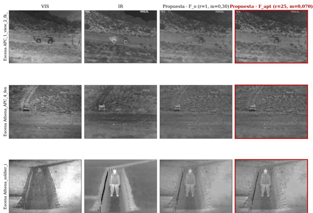
Figura 8. Efecto de la función de aptitud sobre el mismo operador (VIS, IR, F_o , F_{apt} ) en tres escenas del TNO.
