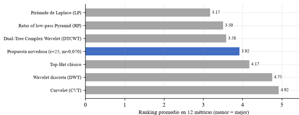
Figura 5. Ranking promedio global de los 7 métodos (12 métricas, dirección respetada); la barra azul es la propuesta.
