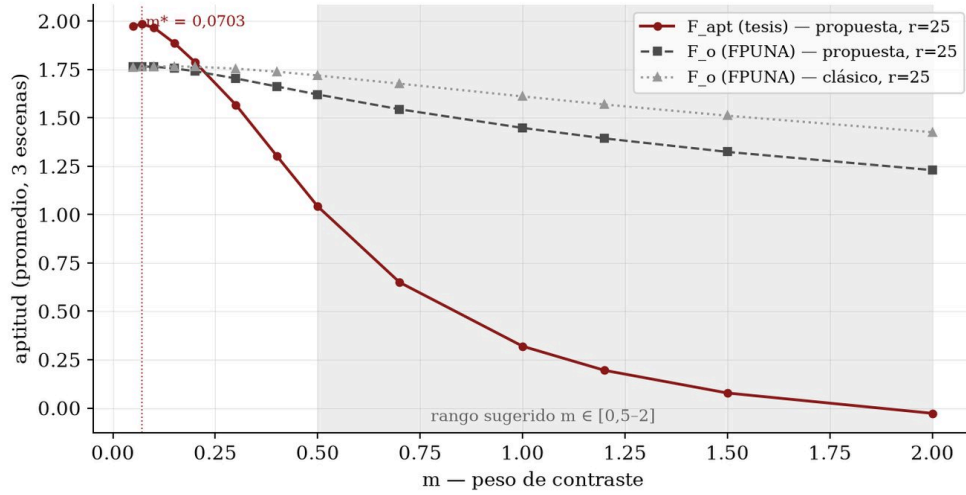
Figura 7. Aptitud en función de m ( r = 25 ), sin restricciones de rango: las tres curvas decrecen monótonamente en [0,5-2] , y el máximo real de F_o sobre la propuesta coincide con nuestro óptimo ( m \approx 0,07 ).
