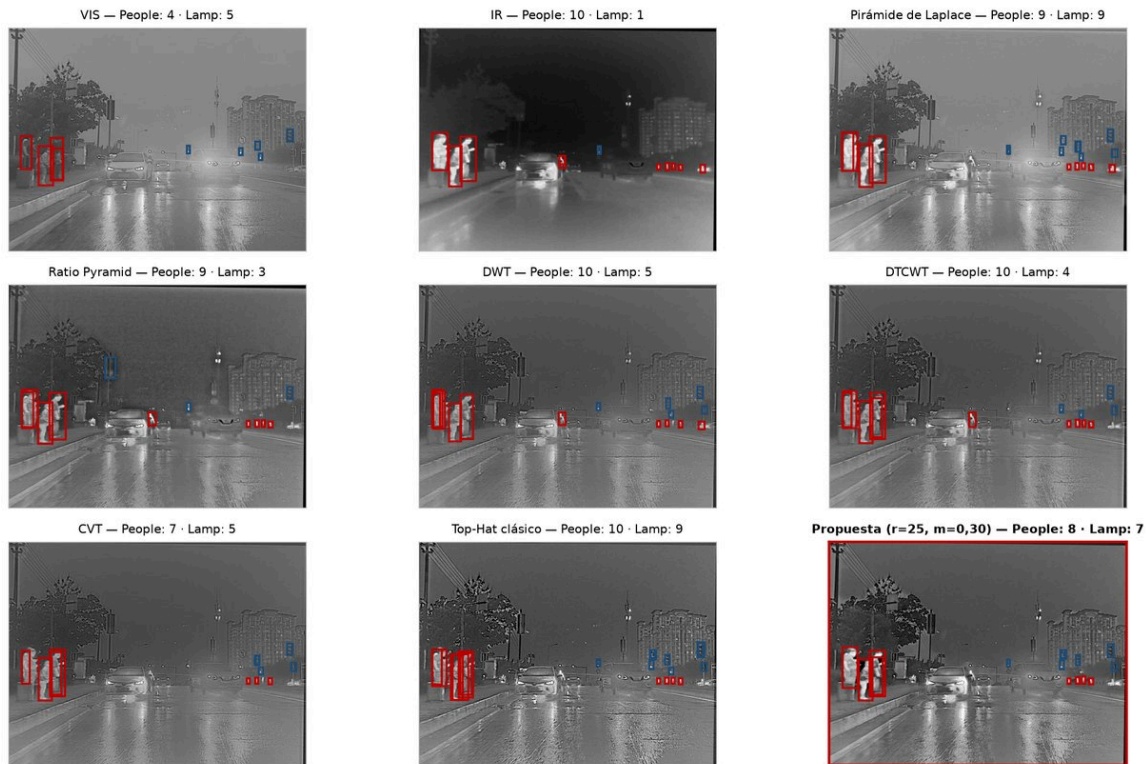
Figura 8. M3FD, escena 00231: detecciones del modelo único VIS+IR sobre cada entrada. People en granate, Lamp en azul, umbral de confianza 0,30. Verdad de campo: 12 personas y 5 luces.
