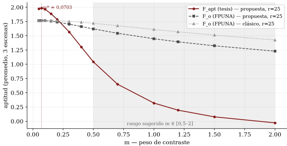
Figura 12. Aptitud en función del peso de contraste m ( r = 25 ), sin restricciones de rango: F_{apt} de la tesis y F_o del trabajo de referencia sobre ambos operadores.
