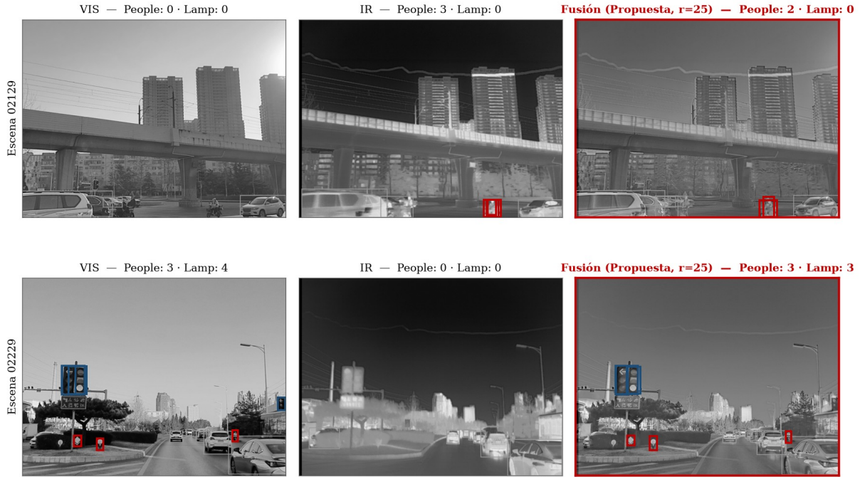
Figura 9. Detecciones del modelo único VIS+IR en dos escenas de la validación de M3FD (personas en recuadro granate, luces en azul): en la escena superior el visible no detecta ninguna persona y la fusión las recupera; en la inferior el infrarrojo no detecta ninguna luz y la fusión las recupera.
