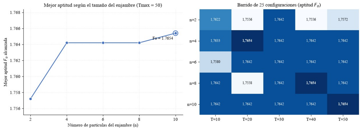
Figura 11. Convergencia del PSO según el número de partículas (izq.) y aptitud del barrido de configuraciones (der.), sobre tres escenas representativas.
