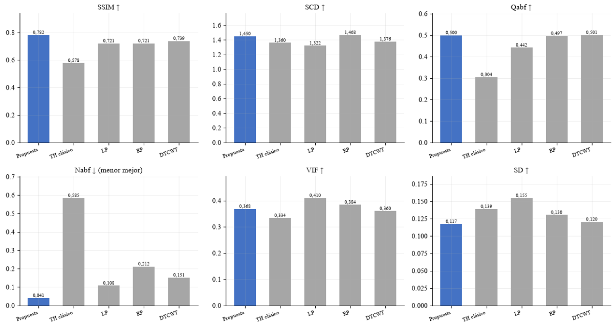
Figura 10. Propuesta Novedosa (PSO: r = 25 , m = 0,070 ) frente a la metodología clásica Top-Hat y al estado del arte en las métricas estándar de calidad.
