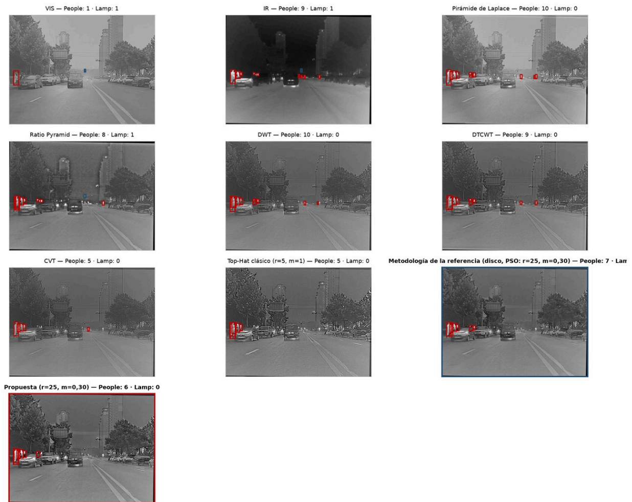
Figura 12. M3FD, escena 00147: detecciones del modelo único VIS+IR sobre las 10 entradas. People en granate, Lamp en azul, umbral de confianza 0,30. Verdad de campo: 12 personas y 1 luz.
