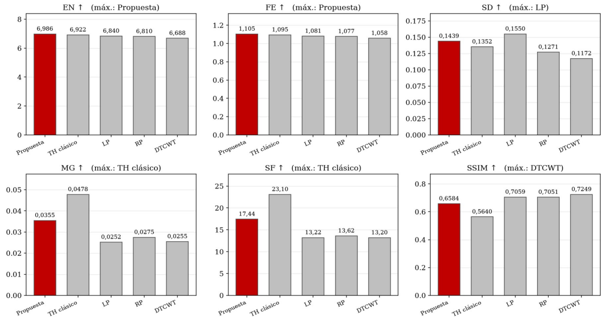
Figura 10. Propuesta Novedosa (PSO: r = 25 , m = 0,30 ) frente a la metodología clásica Top-Hat y a tres métodos del estado del arte en las cinco métricas de actividad e información de la Tabla 10 (EN, FE, SD, MG, SF) y en la similitud estructural, donde el operador cede.
