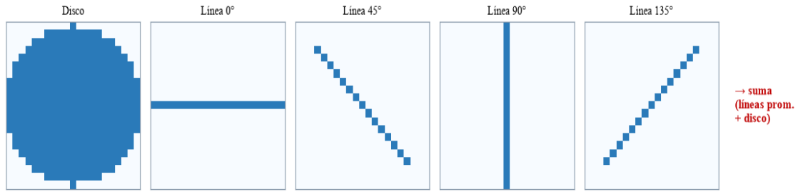
Figura 3. Banco de cinco elementos estructurantes (un disco y cuatro líneas): las respuestas lineales promediadas se suman a la del disco.
