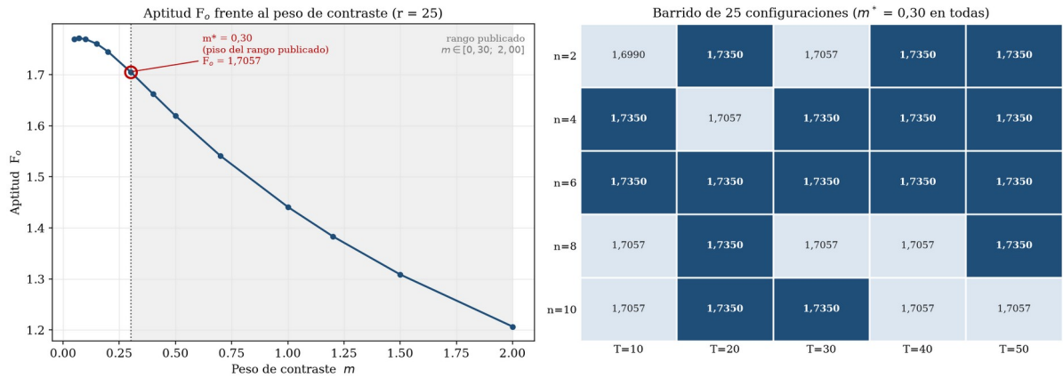
Figura 11. Aptitud F_o en función del peso de contraste con el radio fijo en r = 25 (izq.) y mejor aptitud alcanzada por cada combinación de partículas e iteraciones del barrido (der.), sobre tres escenas representativas. La aptitud decrece de forma monótona a partir de valores pequeños de m , de modo que el óptimo se sitúa en el piso del rango publicado.
