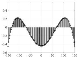
图 5: 最优抛物面与基准球面的偏移量
