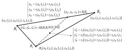
图 9: 反馈面板三角形区域示意图
