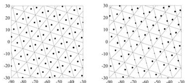
图 11: 在相同区间下, 工作状态(左)与基准态(右)纹理对比
