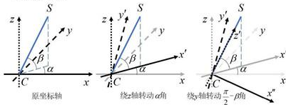
图 6：坐标系旋转示意图
