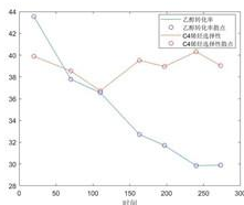
图 4 乙醇转化率与 C4 选择性散点图
