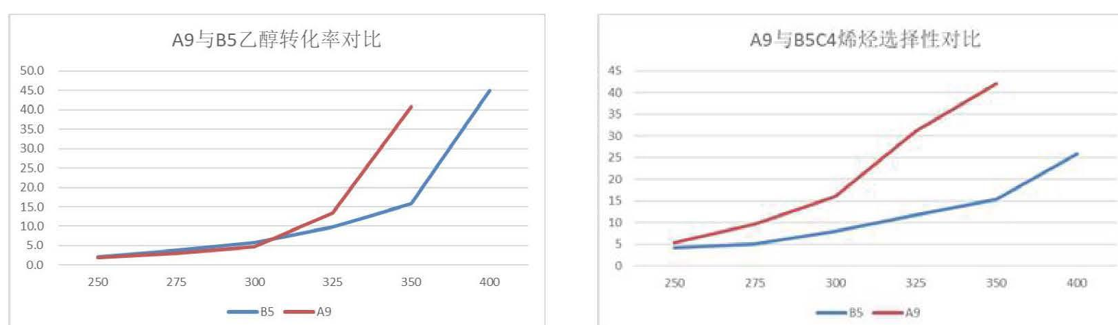
图 8 A9 与 B5 对比图
