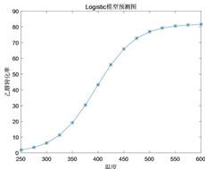
图 3 A1 组的乙醇转化率趋势预测图
