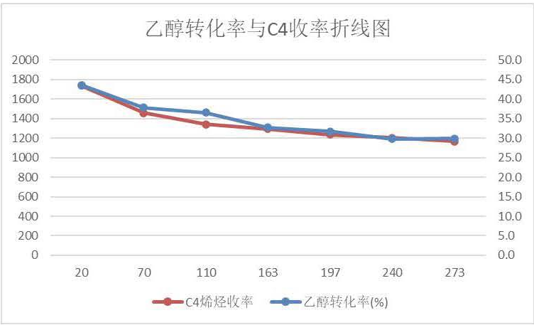
图 6 乙醇转化率与 C4 收率折线图
