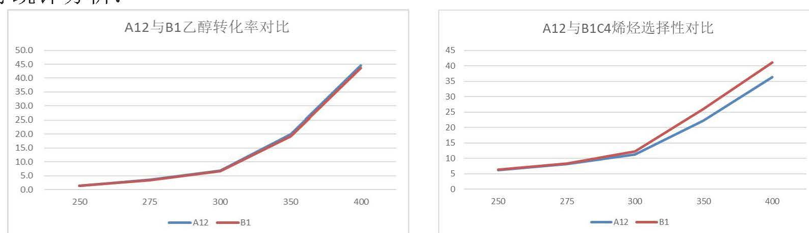
图 7 A12 与 B1 对比图
