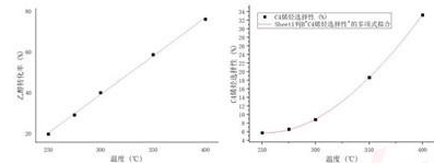
A8: 50mg 1wt%Co/SiO 2 - 50mg HAP-乙醇浓度 0.9ml/min
