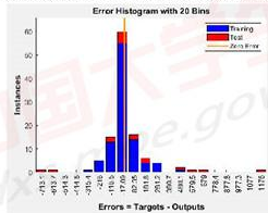
图 5.4-5: 训练数据的历史残差图
