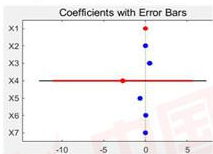
图 5.3-6: y_1^* 带误差条的系数
