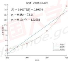
图 5.1-5 B1 组直线拟合与指数拟合对比图
