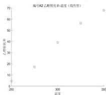
图 5.1-1 线性增长型散点图
