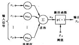
图 5.4-1：人工神经网络基本单元的神经模型
