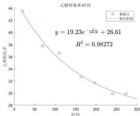
图 5.2-1 乙醇转化率随时间呈指数衰减特征
