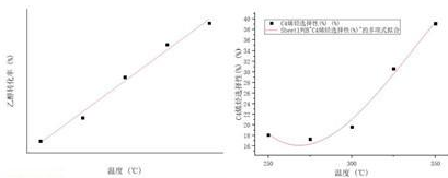
A3: 200mg 1wt%Co/SiO 2 - 200mg HAP-乙醇浓度 0.9ml/min
