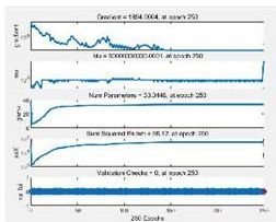
图 5.4-4: 训练数据梯度与均方误差变化图
