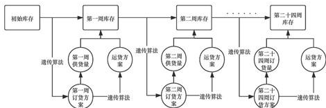
图 2：问题二的多目标规划模型
