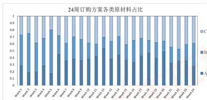
图 7：24 周订购方案各类原材料占比
