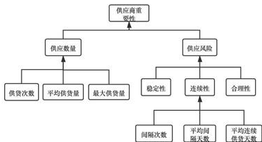
图 1：问题一多指标评价模型
