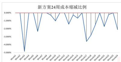
图 14: 新方案 24 周成本缩减比例
