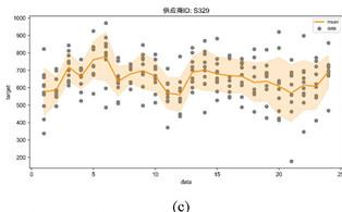
图 4: 以 24 周为周期的历史供货情况 (S080 为(a)、S282 为(b)、S329 为(c))
