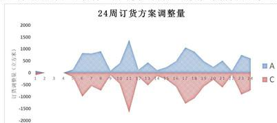
图 13: 24 周订货方案调整量
