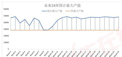
图 15: 未来 24 周预计最大产能
