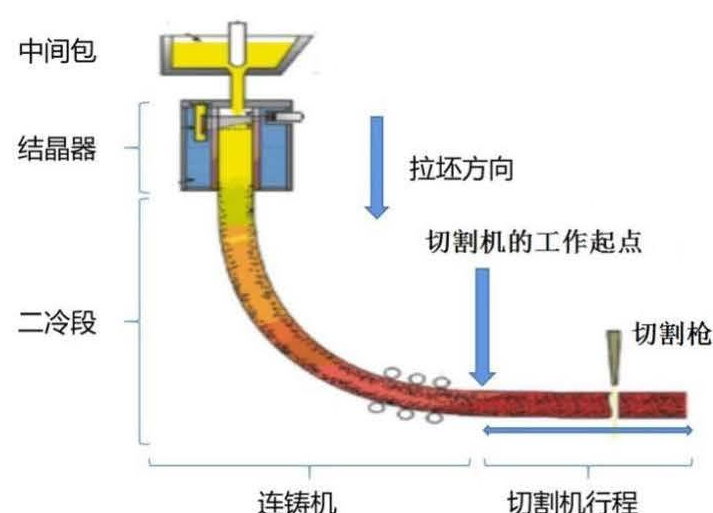
图 1 连铸工艺的示意图
