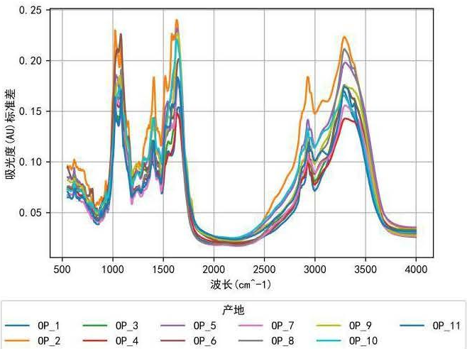
图 5-2 不同产地药材光谱数据标准差曲线
