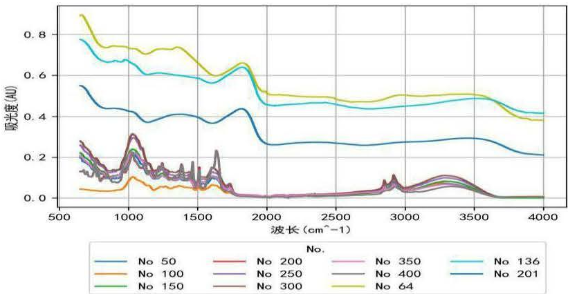
图 4-1 部分药材的中红外光谱数据示意图
