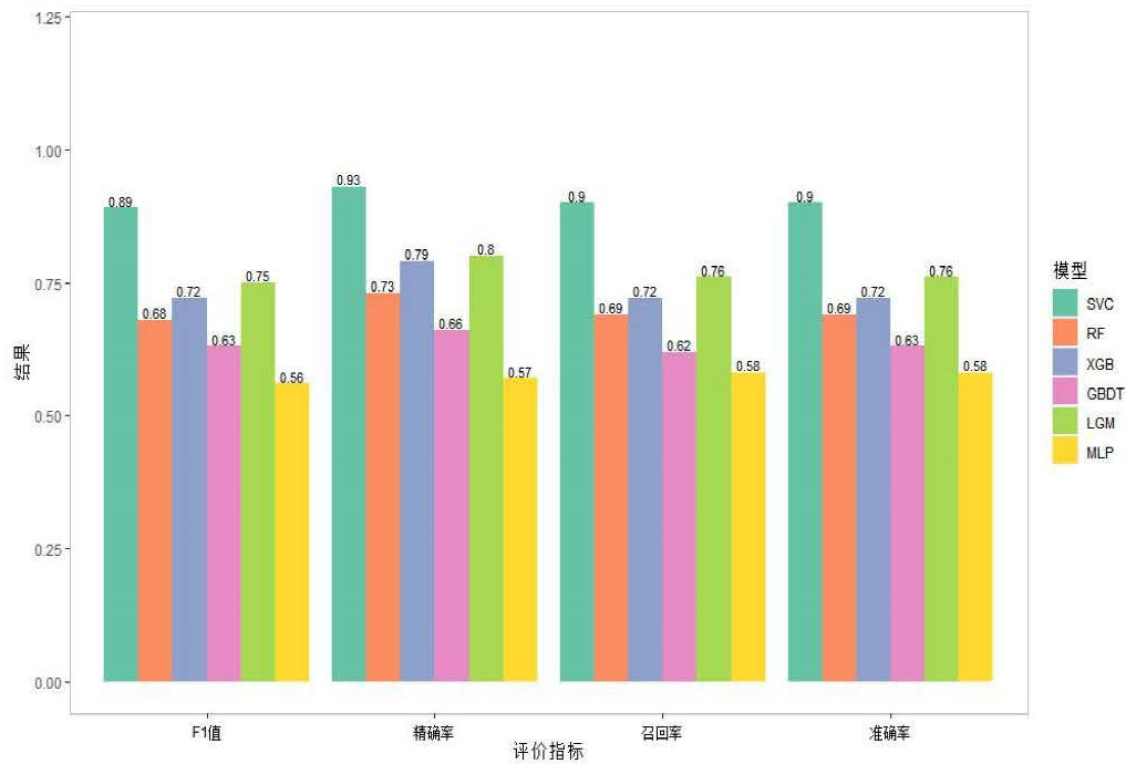
图 6-1 原始数据模型比较
