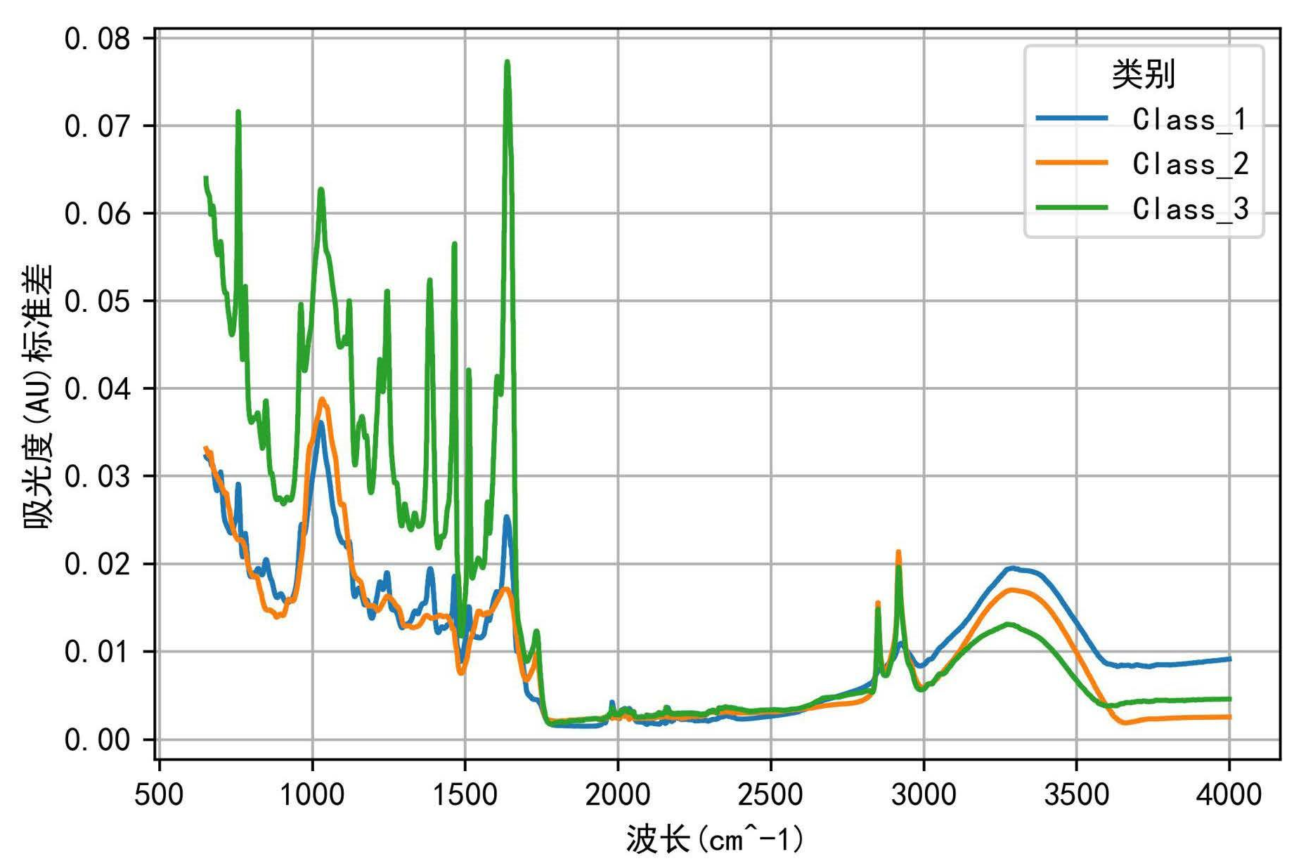
图 4-25 不同种类药材光谱数据标准差曲线
