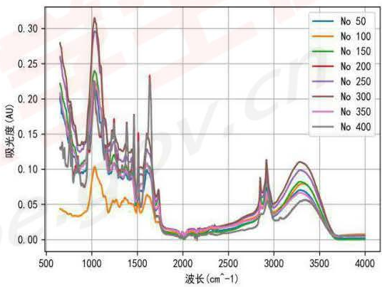
图 4-3. 不同类别药材光谱数据示意图
