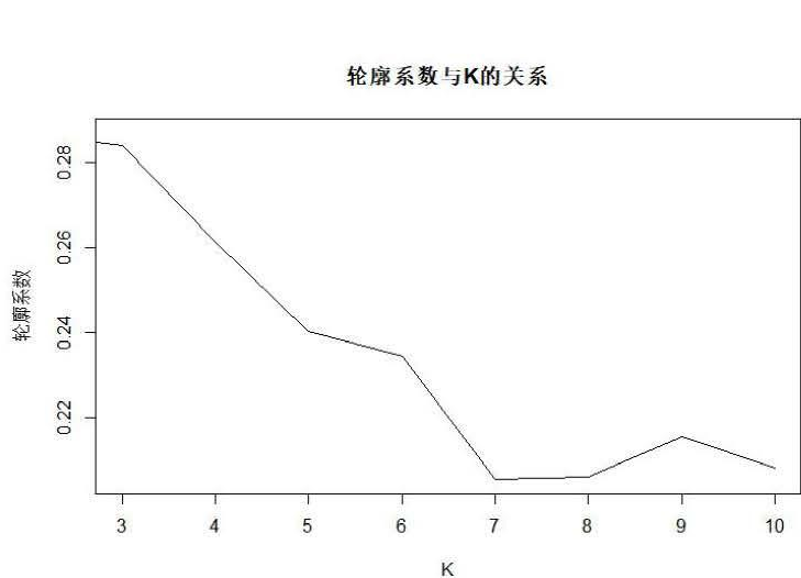
图 4-14.平均轮廓法确定聚类数
