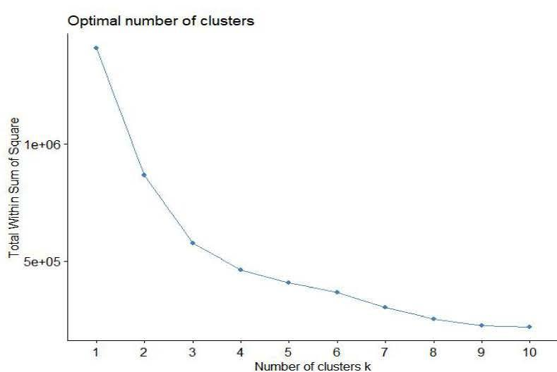
图 4-4.肘部法则确定聚类数
