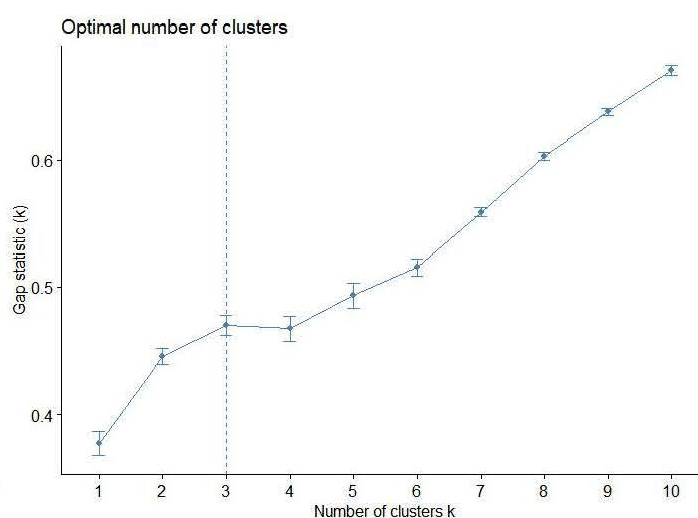
图 4-5.间隔统计量确定聚类数
