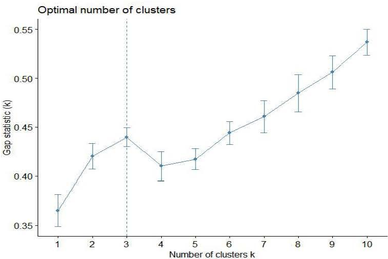
图 4-9.间隔统计量确定聚类数
