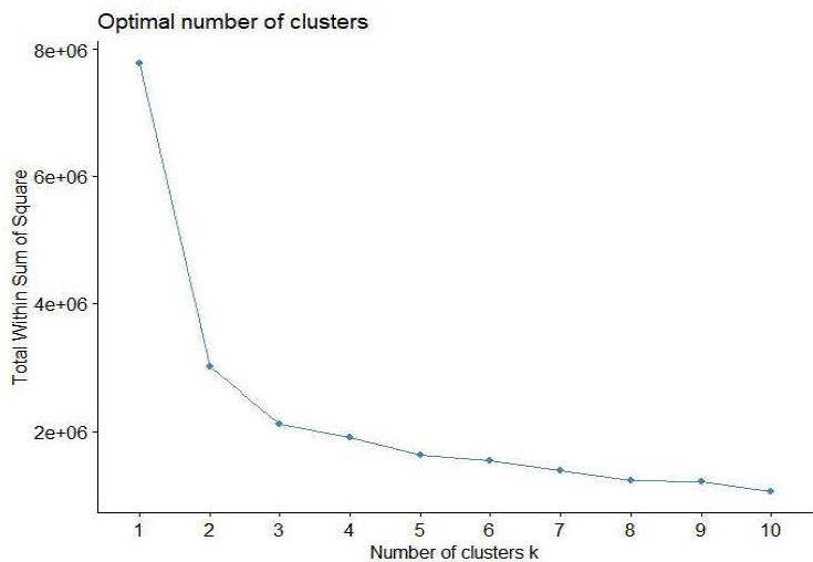
图 4-8.肘部法则确定聚类数
