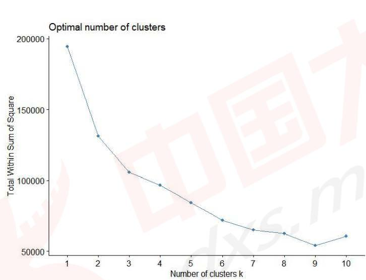
图 4-16.肘部法则确定聚类数
