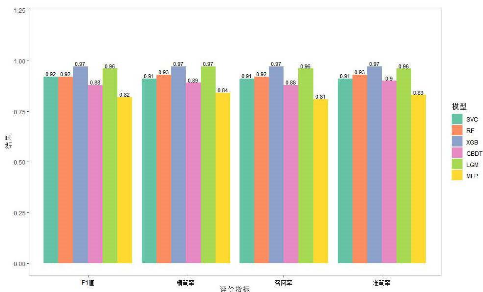
图 5-2 波段-20 数据集模型比较
