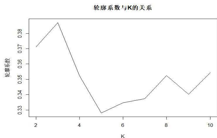
图 4-6.平均轮廓法确定聚类数
