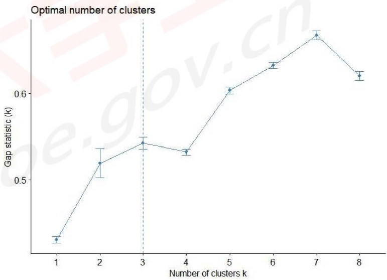
图 4-17.间隔统计量确定聚类数
