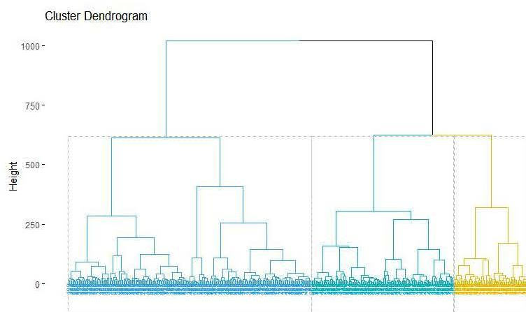
图 4-20. Ward 聚类谱系图
