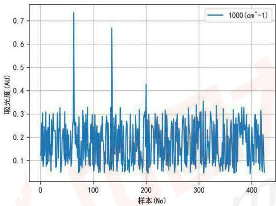
图 4-2. 同一波数对应吸光度数据示意图
