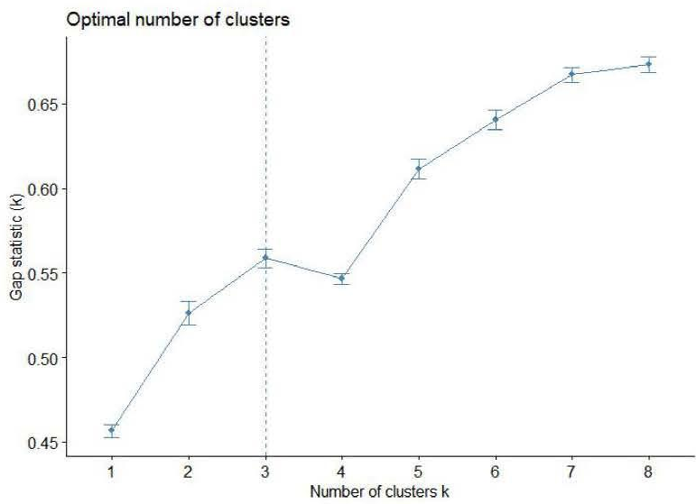
图 4-13.间隔统计量确定聚类数
