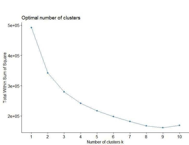
图 4-12.肘部法则确定聚类数
