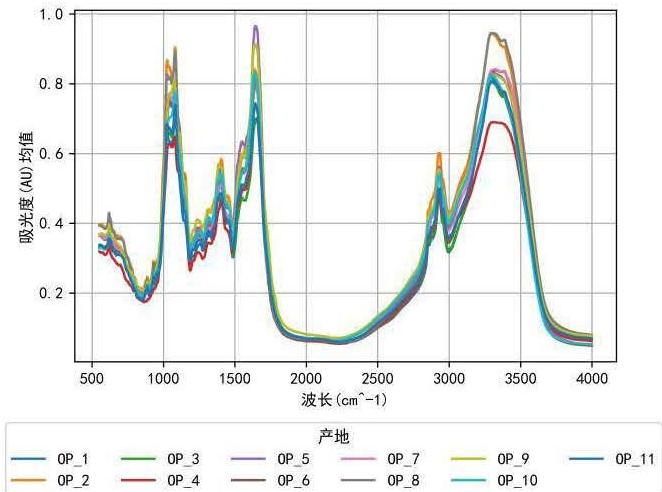
图 5-1 不同产地药材光谱数据均值曲线
