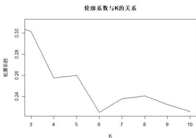
图 4-18.平均轮廓法确定聚类数
