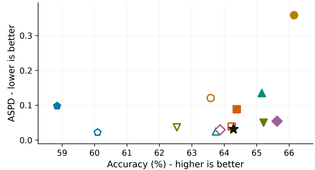
(d) COMPAS: ACC vs ASPD
