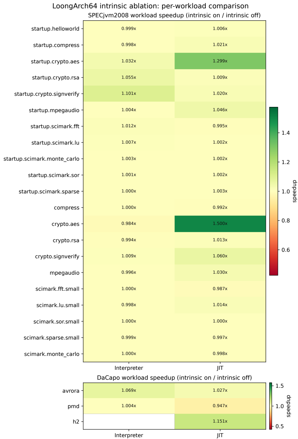
图 5.5 LoongArch64 Intrinsic 开关消融实验的逐工作负载收益热力图
