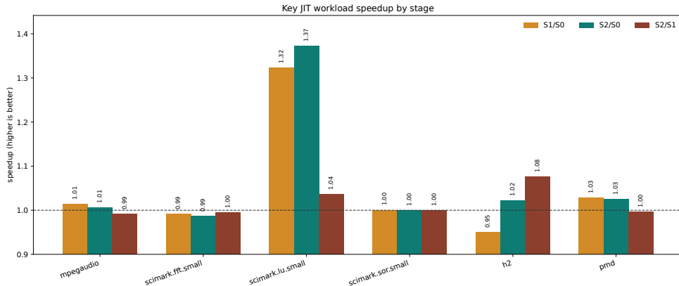
图 5.1 完整 SIMD 覆盖候选版在关键工作负载上的相对收益
