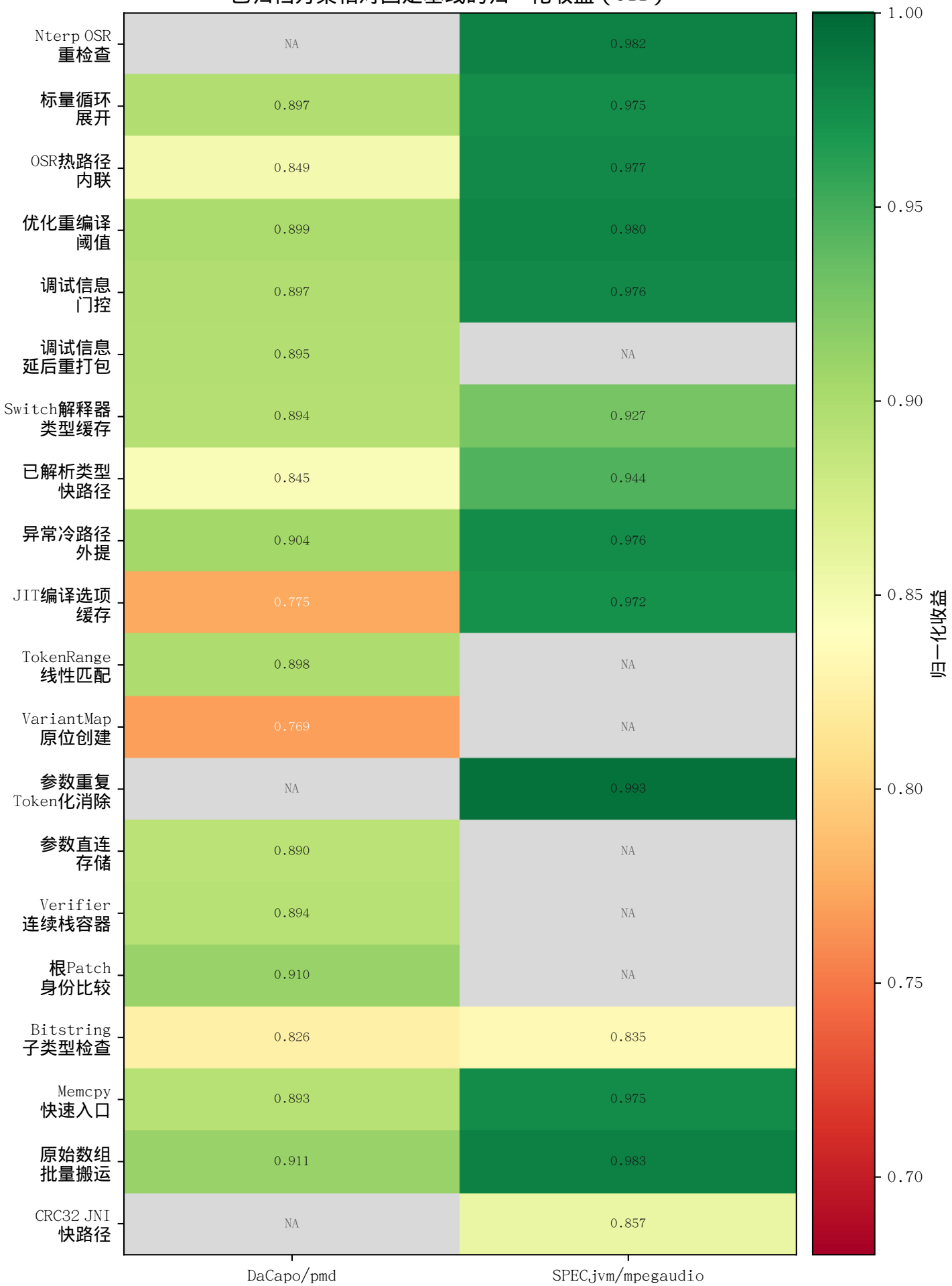
已归档方案相对固定基线的归一化收益 (JIT)
