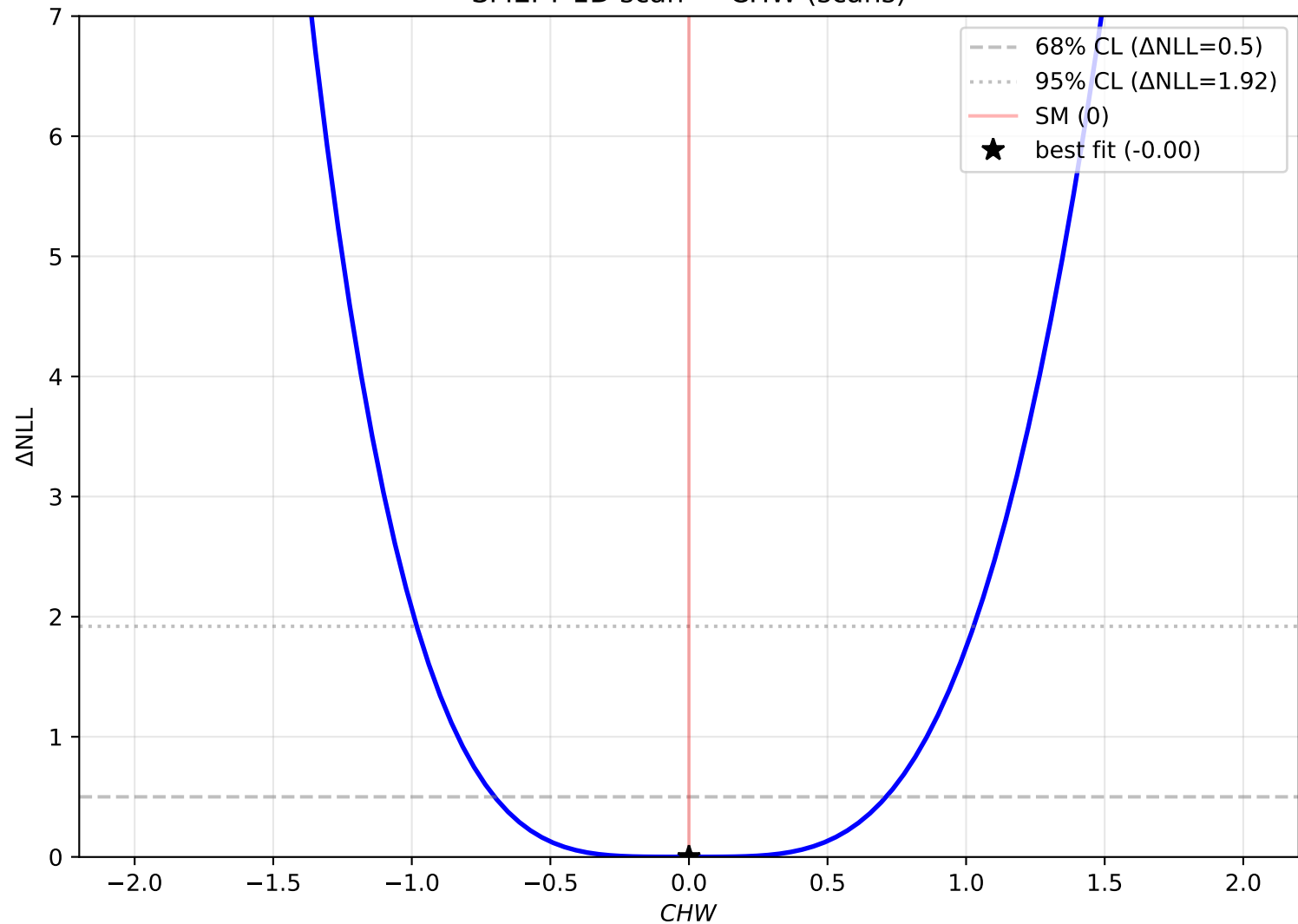
SMEFT 1D scan — CHW (scans)
