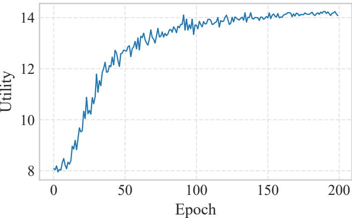
PPO_Convergence
