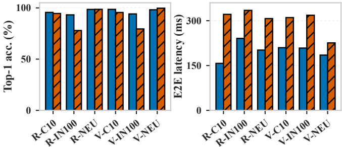
SEAS I-SplitEE
