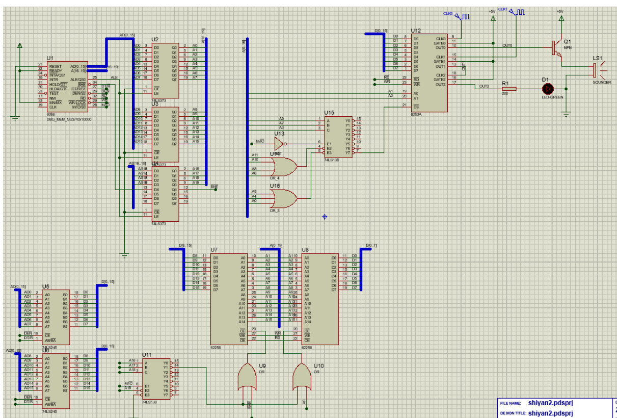
图 5. Proteus 实验二仿真电路原理图
