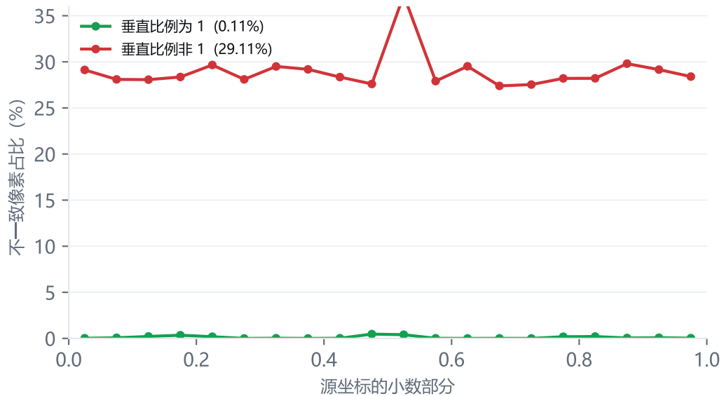
(b) 已交付的 resize vs OpenCV, 135 个尺度
