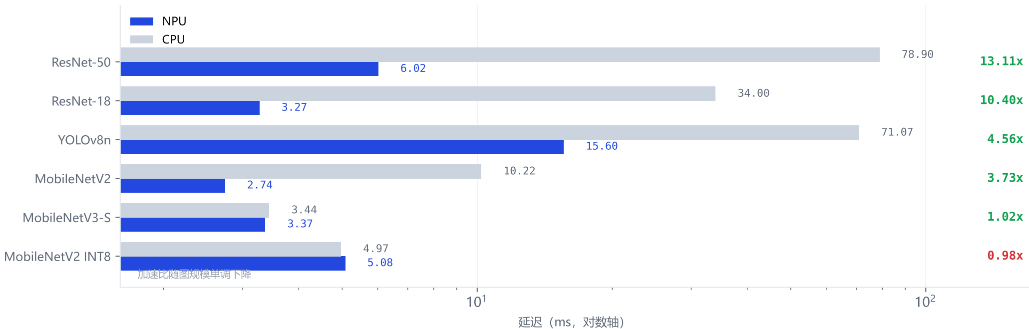
麒麟 8020: NPU 与 CPU 延迟对比 (P50, ms)
