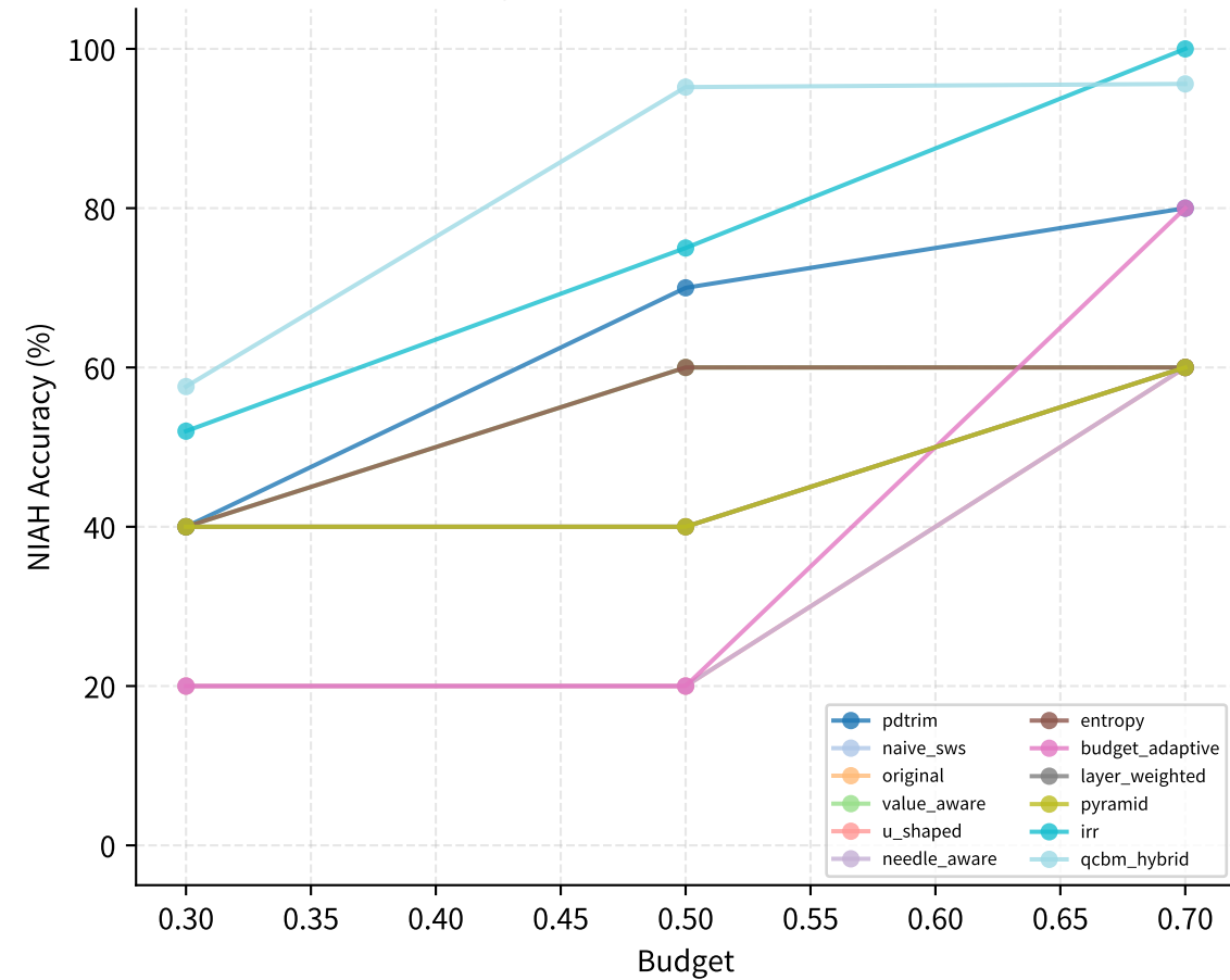
gemma-9b (seq=4096)
