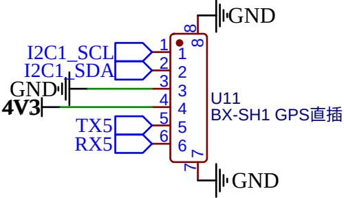
GPS焊盘和GPS直插
