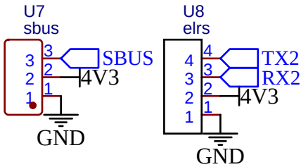
sbus或者串口接收机
