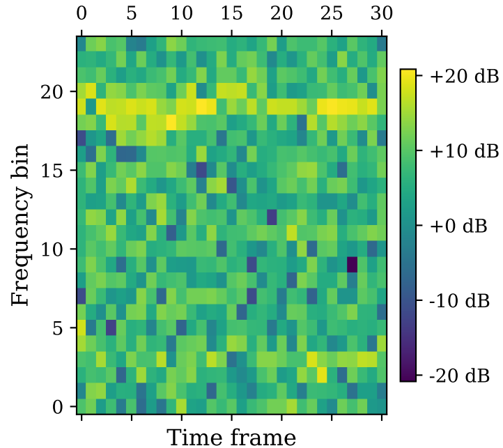
Real Wi-Fi CSI
