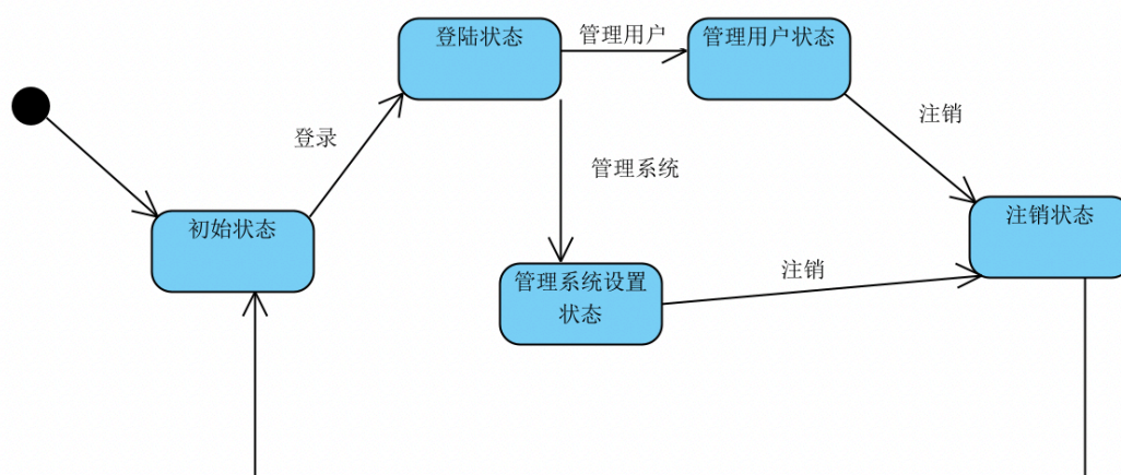
图 5 管理员状态图
