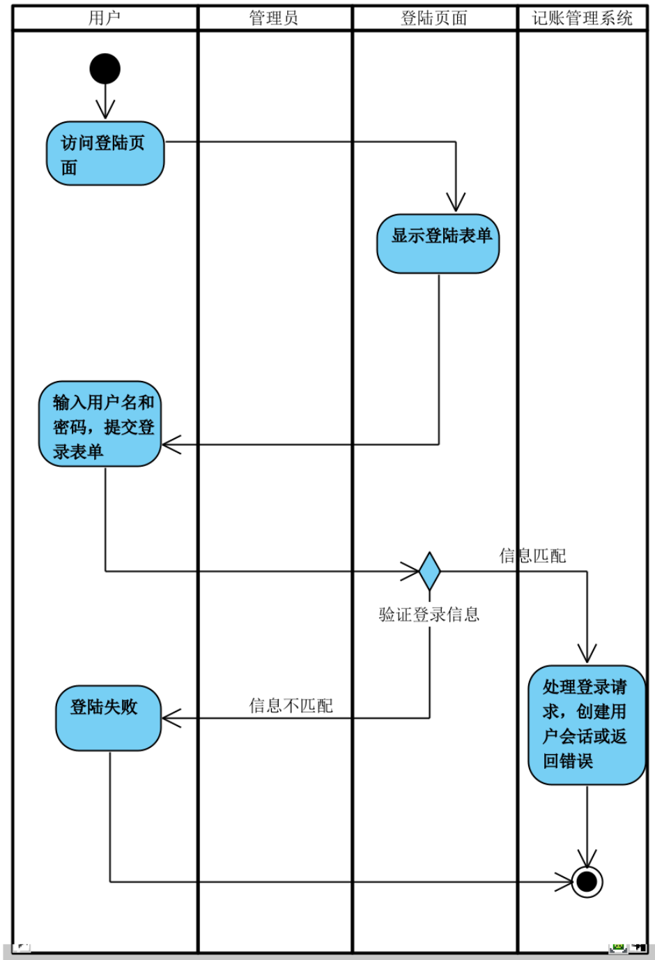
图 1 用户登陆活动图
