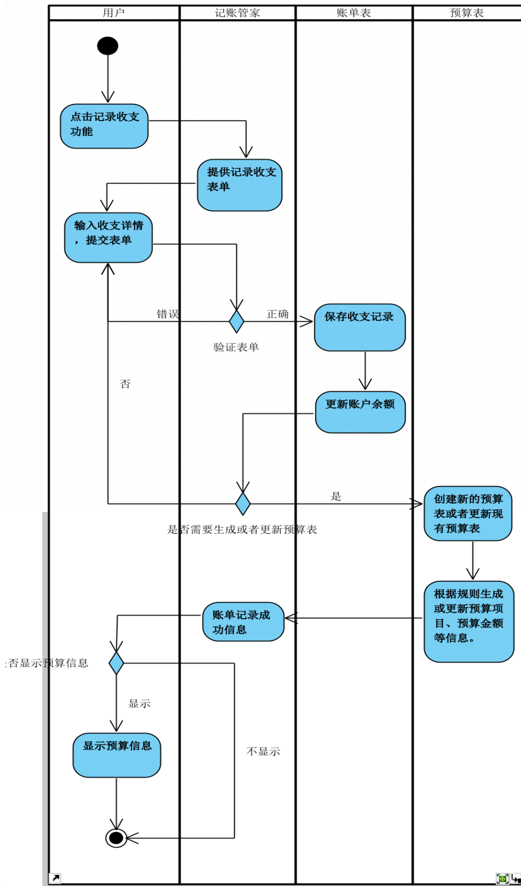
图 2 记录收支活动图
