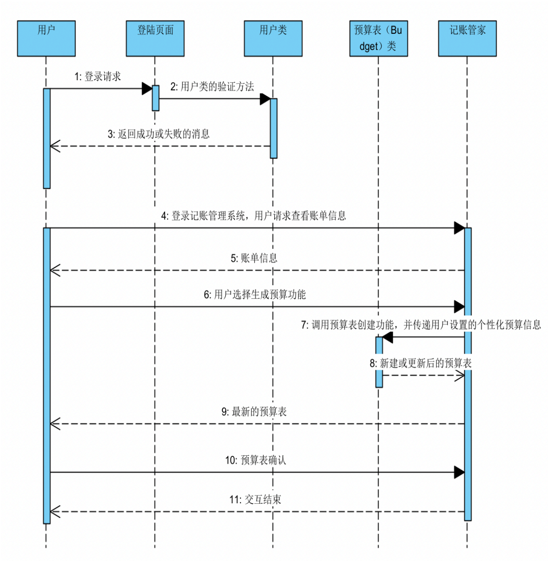
图 3 用户登录、查看账单顺序图
