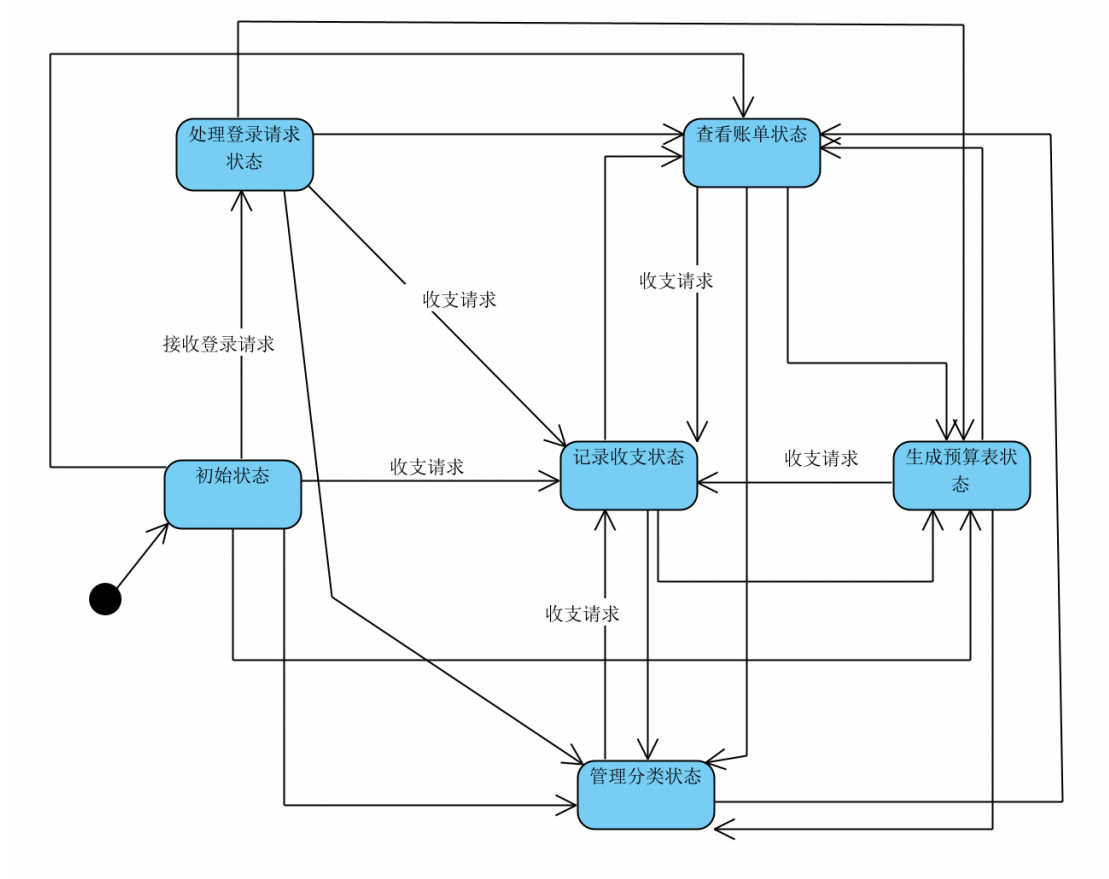
图 6 记账管家状态图
