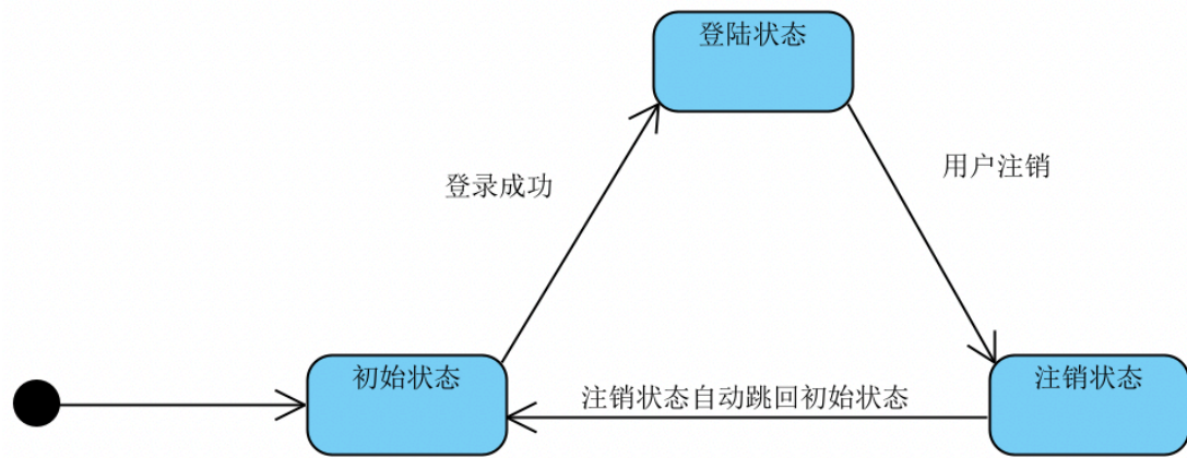
图 4 用户状态图
