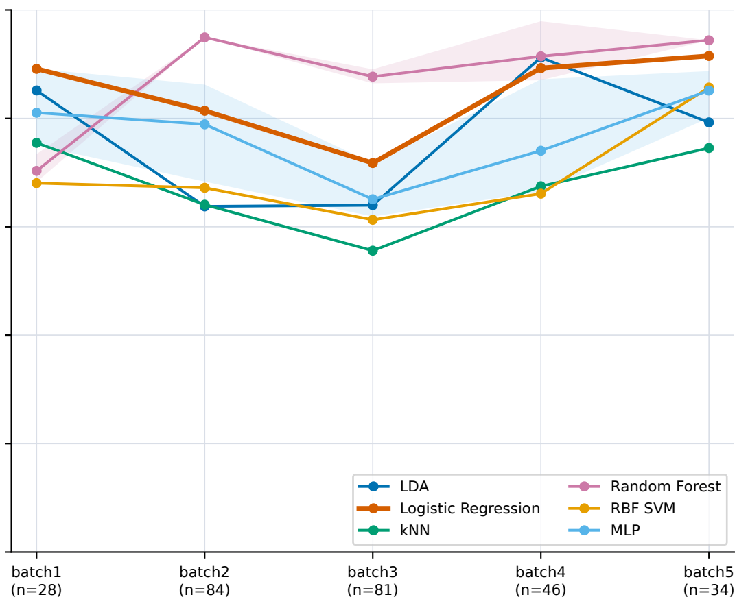
Test macro-F1
