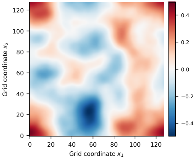
Input vorticity
