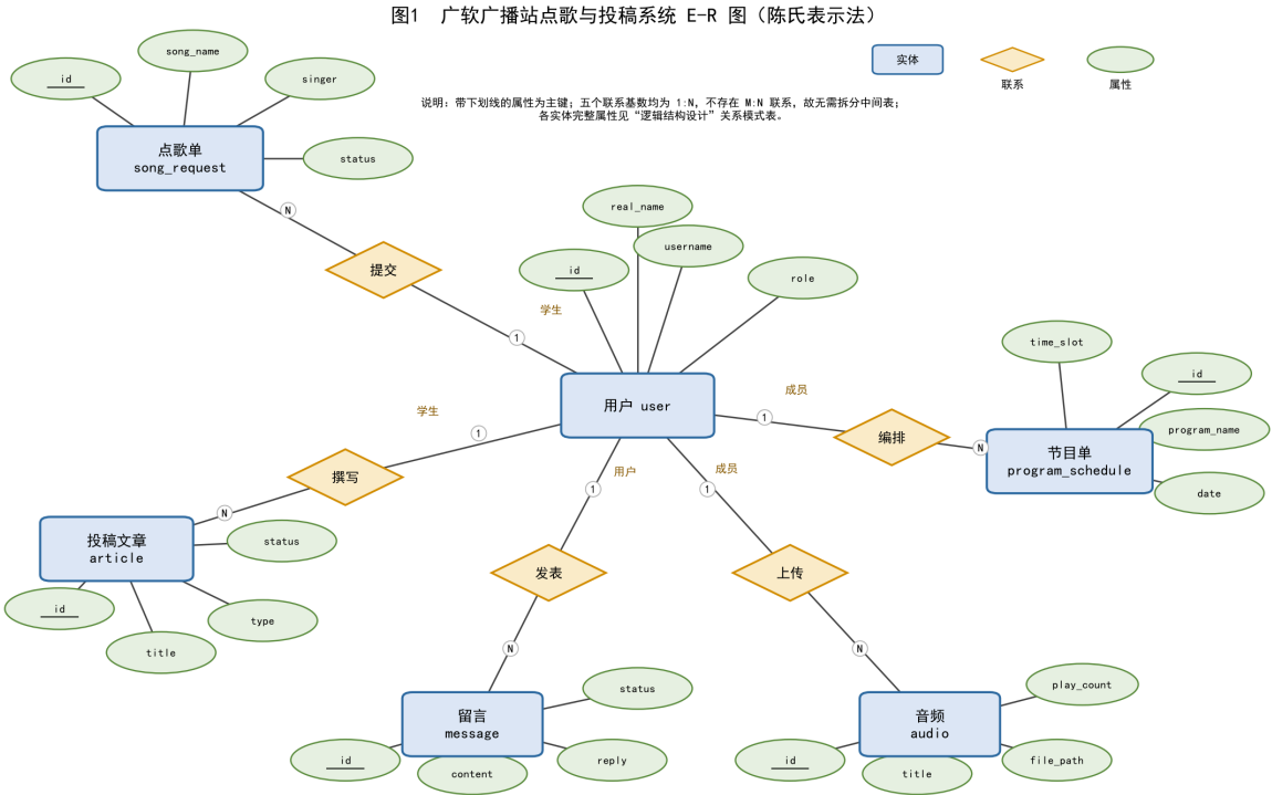
图4-1 系统 E-R 图
