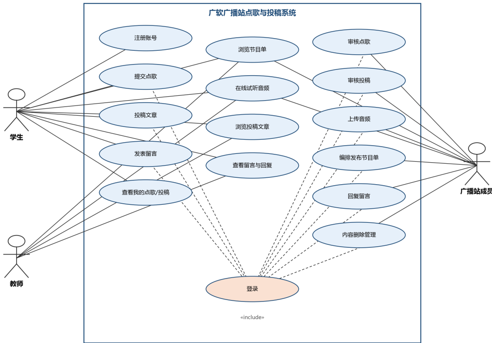
图3-3 系统用例图
