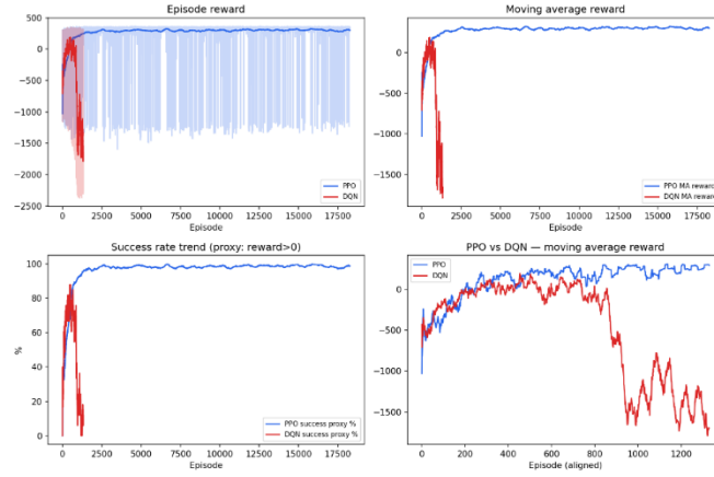
ŞEKİL 5.2.3. PPO ve DQN Eğitim Sürecinde Episode Reward Trend Eğrileri
