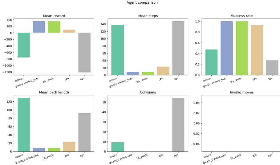
ŞEKİL 5.2.2. PPO ve DQN Algoritmalarının Çoklu Metrik Karşılaştırması
