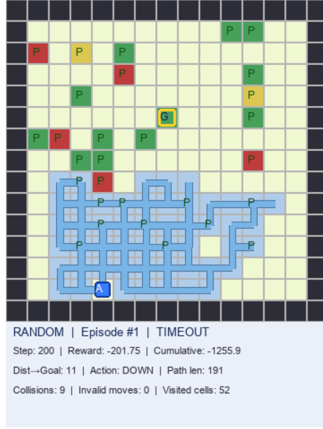
ŞEKİL 5.4.2. Random Baseline Sonucu
