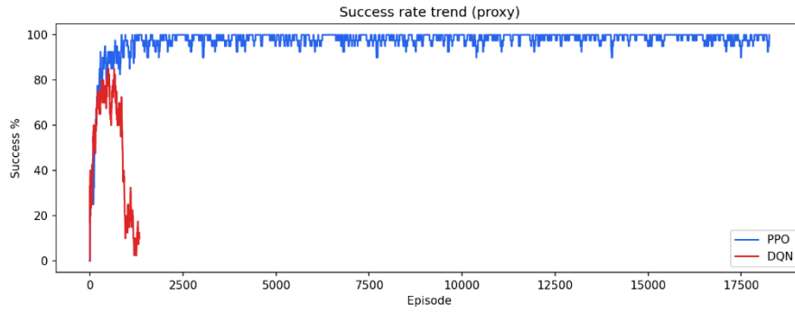
ŞEKİL 5.2.4. Eğitim Sürecinde Başarı Oranı Proxy Trendi (ödül > 0)
