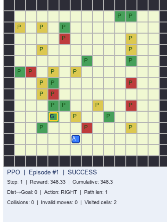
ŞEKİL 5.2.1. PPO Ajanının Hedef Otoparka Ulaşma Performansı
