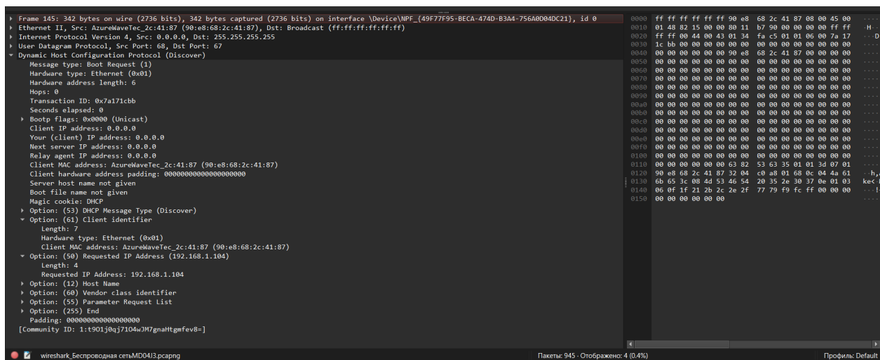
Рисунок 1 — DHCP Discover
