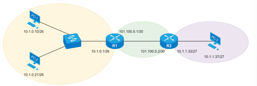
Рисунок 2 — Топология сети
