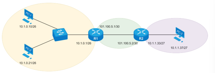
Рисунок 2 — Топология сети
