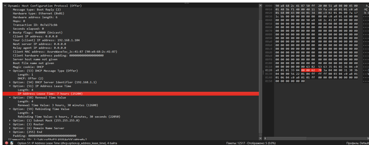
Рисунок 2 — DHCP Offer
