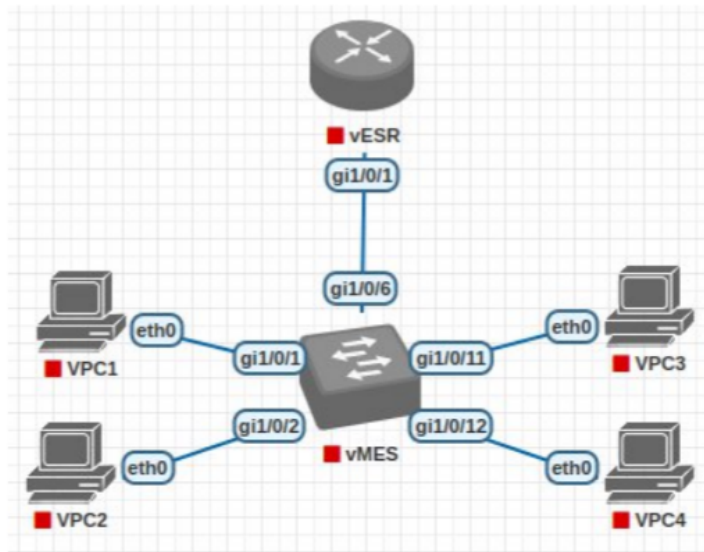
Рисунок 1 — Пример собранной сети
