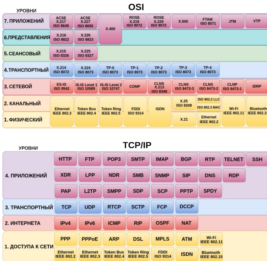
Рисунок 1 — Протоколы OSI и TCP/IP
