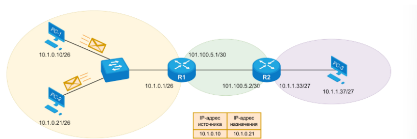
Рисунок 5 — Топология сети
