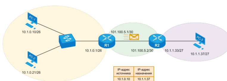
Рисунок 6 — Топология сети
