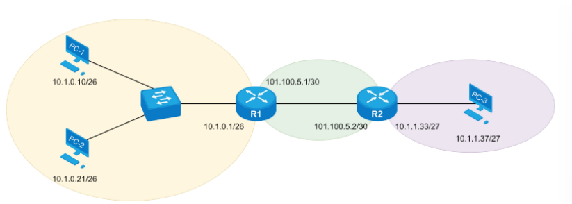
Рисунок 2 — Топология сети
