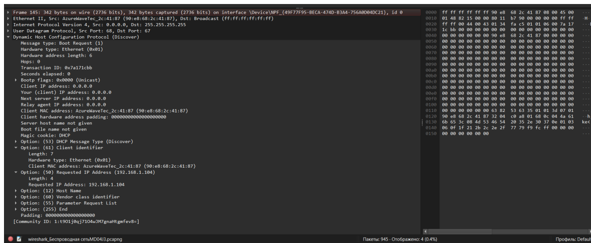
Рисунок 1 — DHCP Discover
