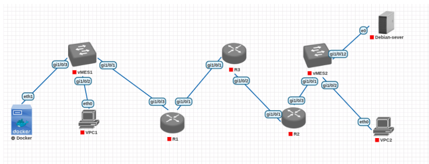
Рисунок 1 — Пример собранной сети
