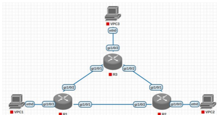
Рисунок 1 — Пример собранной сети
