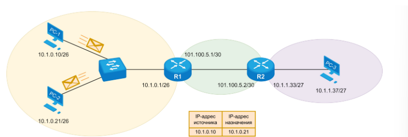
Рисунок 5 — Топология сети
