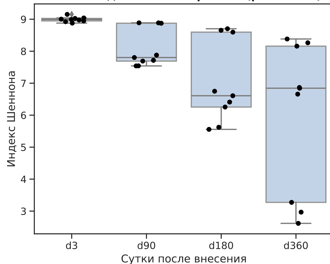
Shannon: динамика во времени (p = 0.0003)
