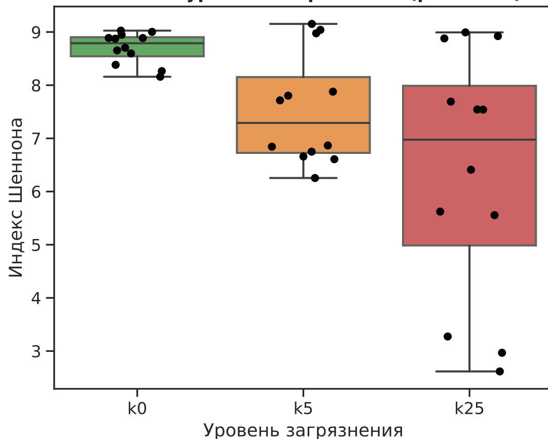
Shannon: уровень загрязнения (p = 0.008)
