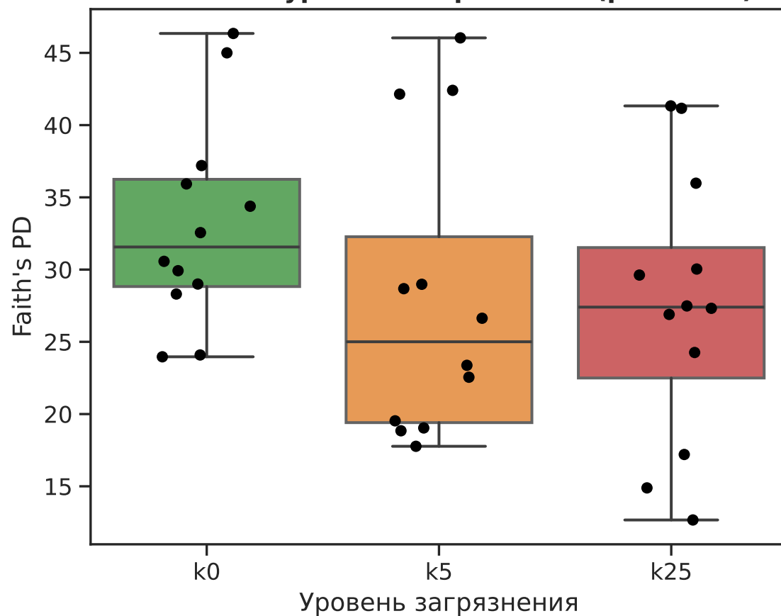
Faith's PD: уровень загрязнения (p = 0.057)
