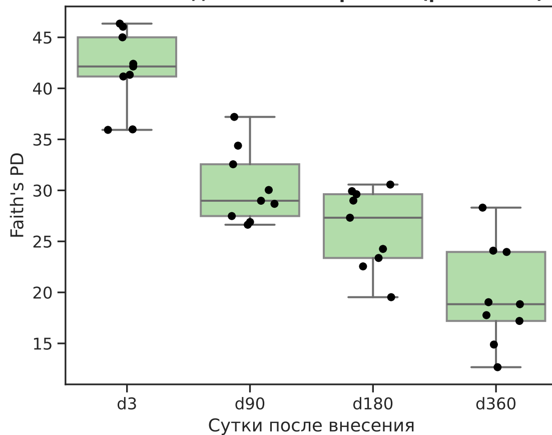
Faith's PD: динамика во времени (p = 0.0003)
