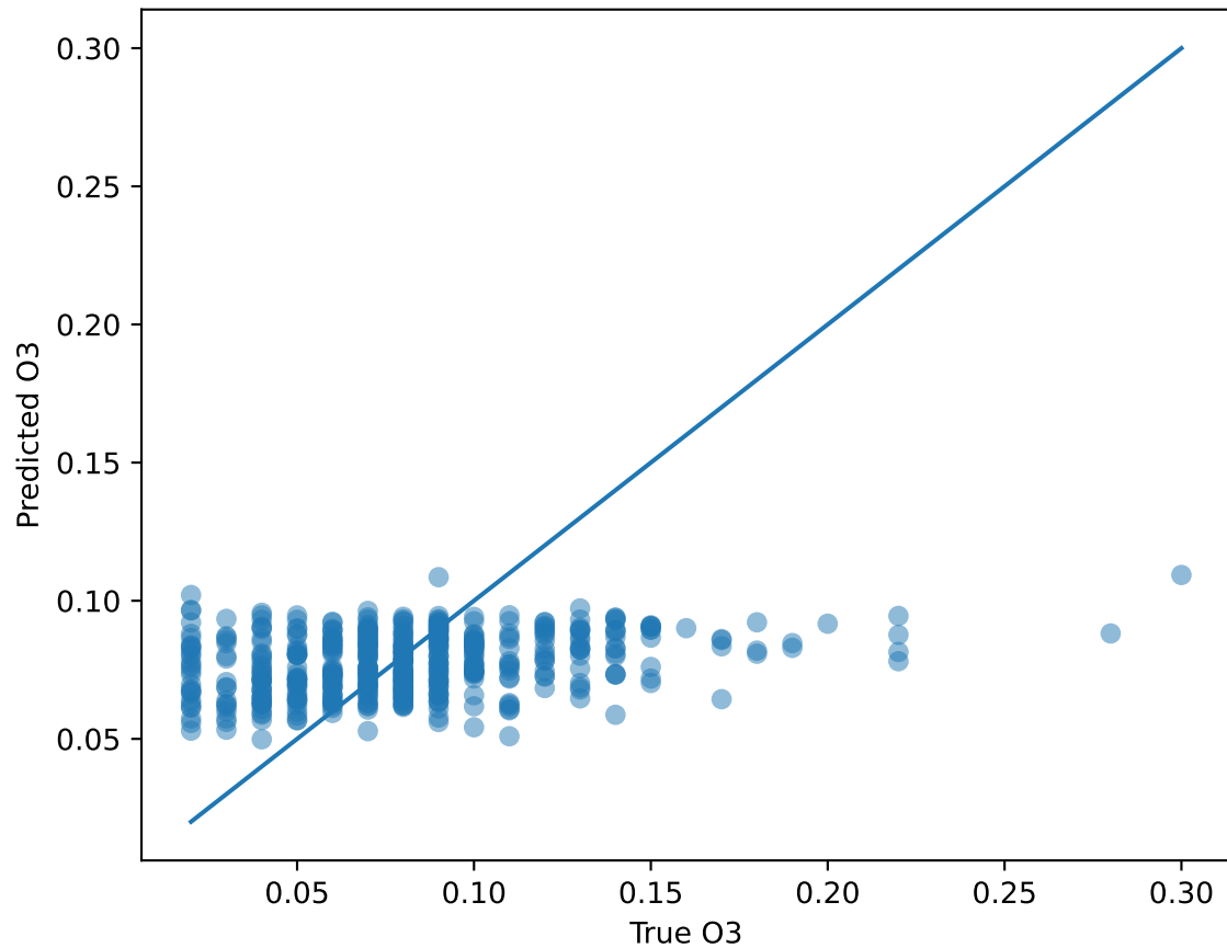
Linear Regression
