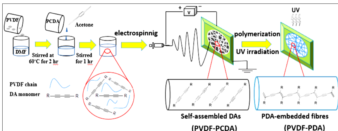
شکل 4-1 طرحواره‌ای از روش تولید نانوالیاف PVDF/PDA [۱۰]
