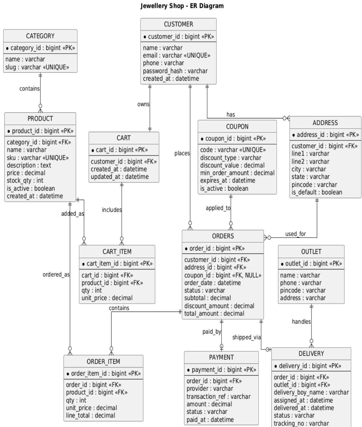
Fig 4.5 ER Diagram
