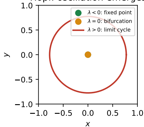
Hopf: oscillation emerges
