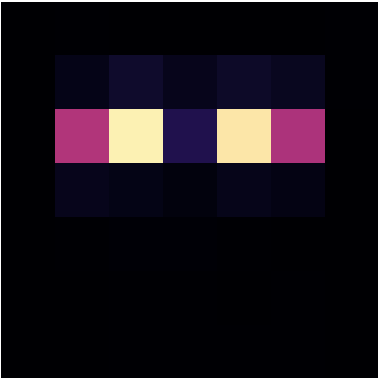
XAI (S4)
