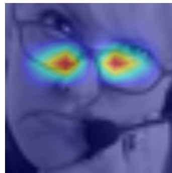
XAI (S4)
