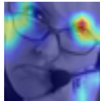
XAI (S5/B1)
