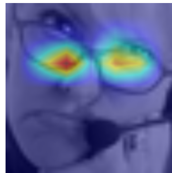
XAI (S4)
