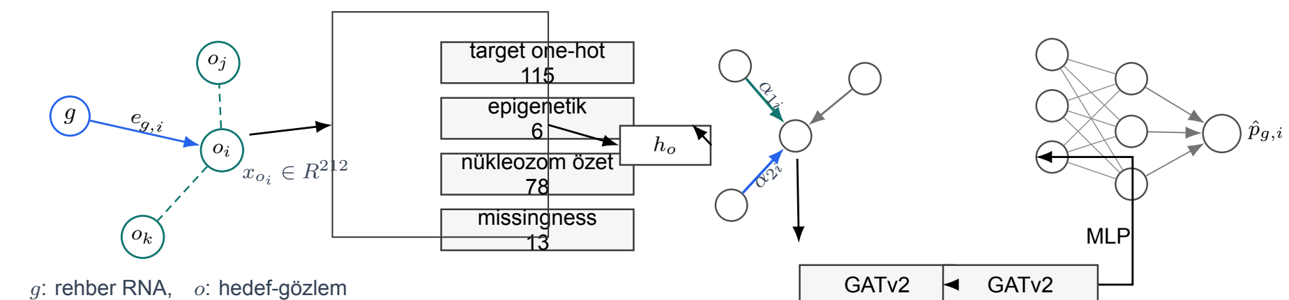
Şekil 1. Ölçülmüş veri sözleşmesi ve kodla uyumlu Graph C/GATv2 akışı: hedef-gözlem düğümü 212 kolonluk bağlamı, candidate edge ise mismatch ve bağlanma enerjisi özelliklerini taşır.
