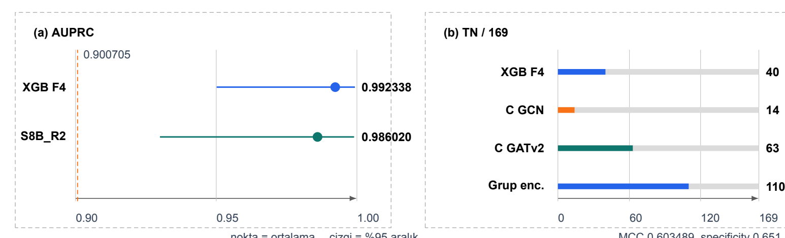
Şekil 3. İki eksenli bulgular: sıralama (AUPRC) ve karar eşiği (MCC/specificity). AUPRC birincil sıralama metriğidir; 0.900705 no-skil PR baseline'dır.
