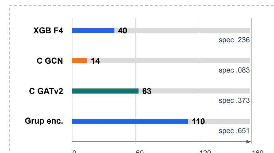
Şekil 4. Karar eşiğinde nadir negatife tanıma: 169 ölçülmüş negatif üzerinden doğru negatif sayıları. Sonuçlar validation-kilitli ve seed/rehber RNA duyarlıdır.
