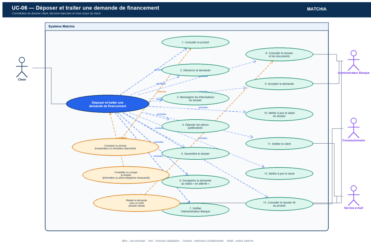
Figure 3.13 — Diagramme de cas d'utilisation détaillé de la demande de financement
