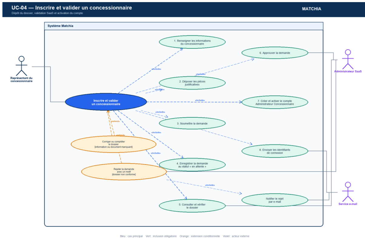
Figure 3.10 — Diagramme de cas d'utilisation détaillé de l'inscription et de la validation d'un concessionnaire
