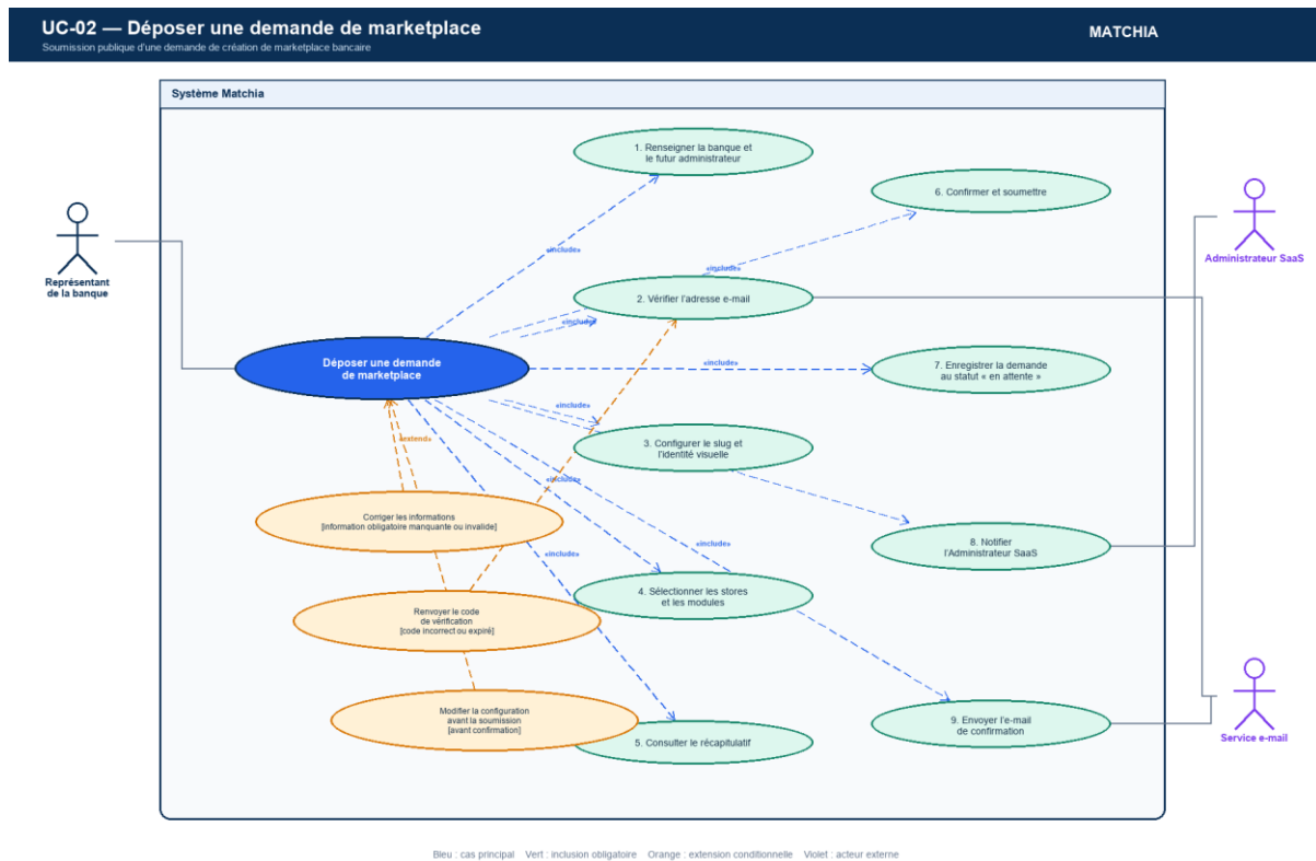
Figure 3.6 — Diagramme de cas d'utilisation détaillé de la demande de création d'une marketplace
