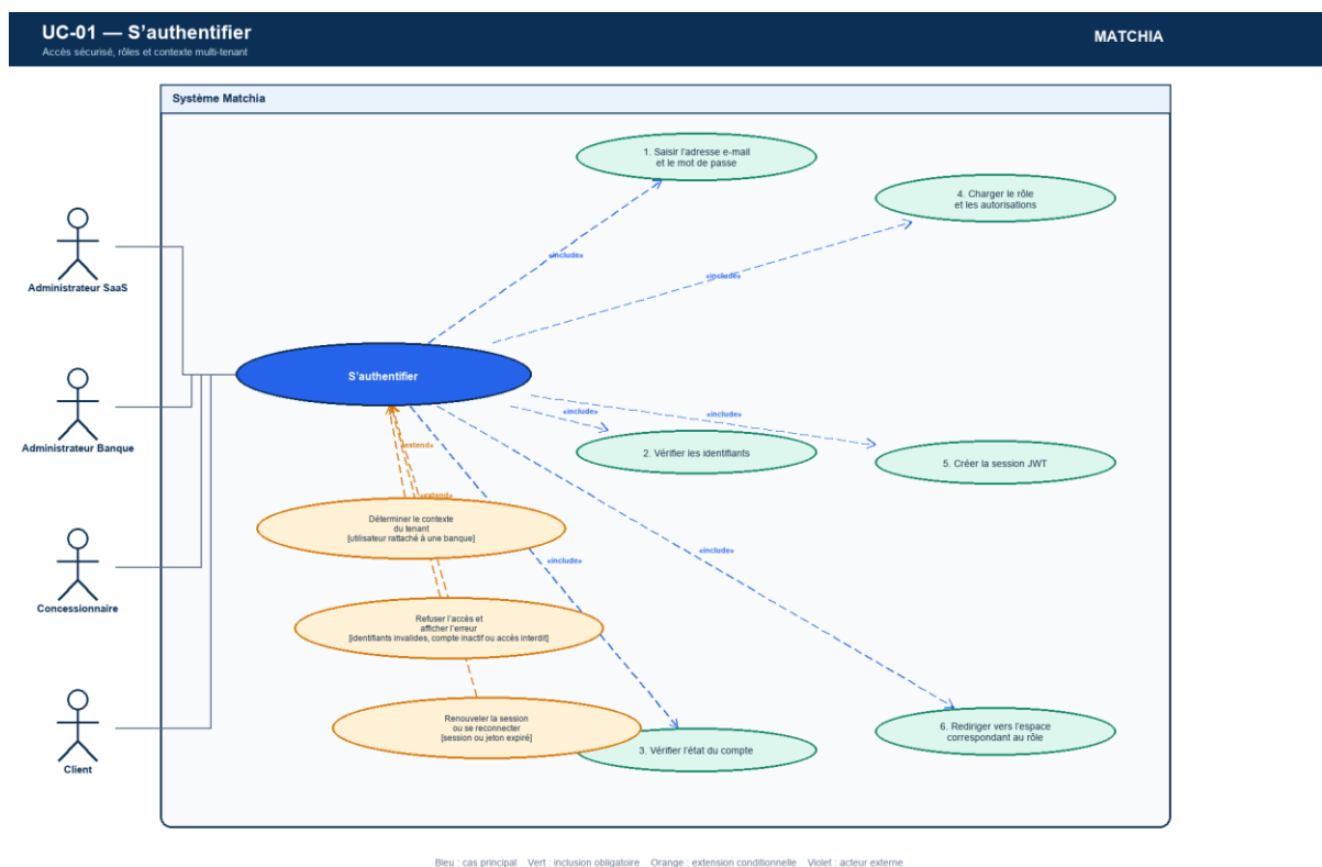
Figure 3.5 — Diagramme de cas d'utilisation détaillé de l'authentification
