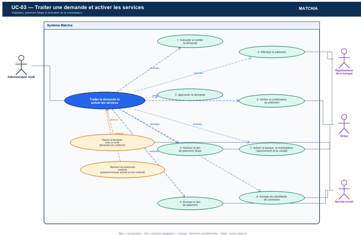
Figure 3.8 — Diagramme de cas d'utilisation détaillé du traitement, du paiement et de l'activation
