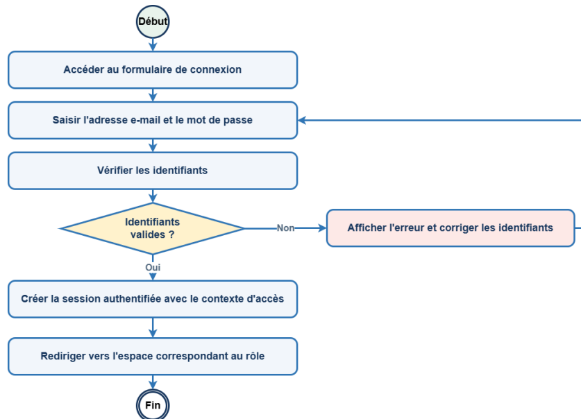
Figure 4.1 — Diagramme d'activité de l'authentification et du contexte d'accès
