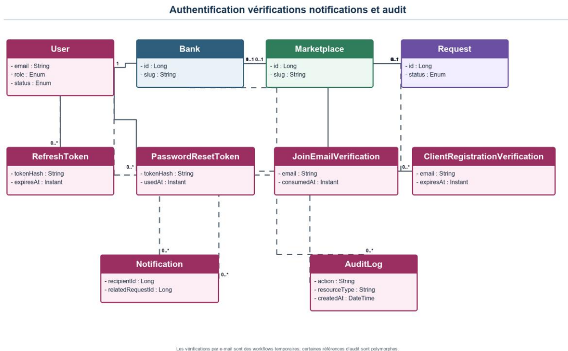
Figure 9 : Authentification, vérifications, notifications et traçabilité
