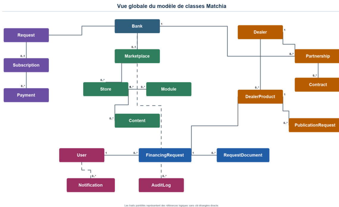
Figure 4 : Vue globale du modèle de classes Matchia
