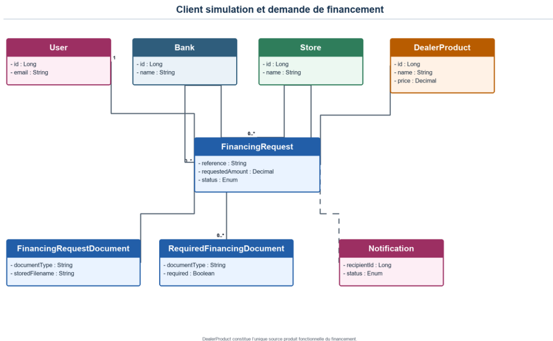
Figure 8 : Client, simulation et traitement d'une demande de financement
